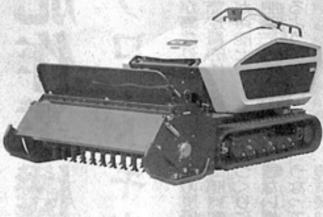
大型草刈機「HM5500」
