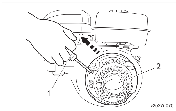
エンジン始動手順_008
