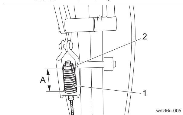
クラッチスプリングの調整_001
