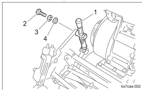
ベッドナイフ台の取り付け_002
