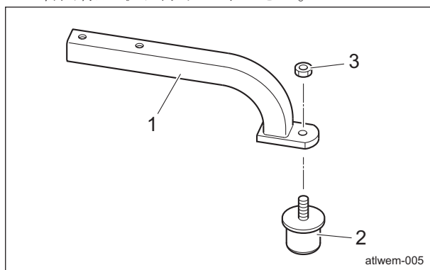
コンツアデッキの取り付け方法_005
