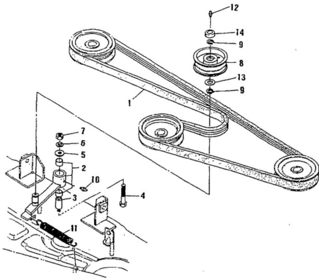
Vベルト、テンション V-BELT, TENSION
