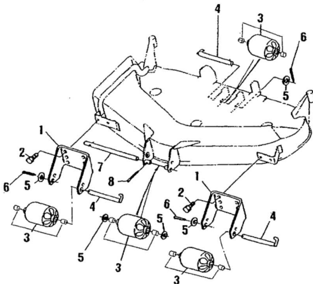
ローラ :フロント & リヤ ROLLER ;FRONTT & REAR
