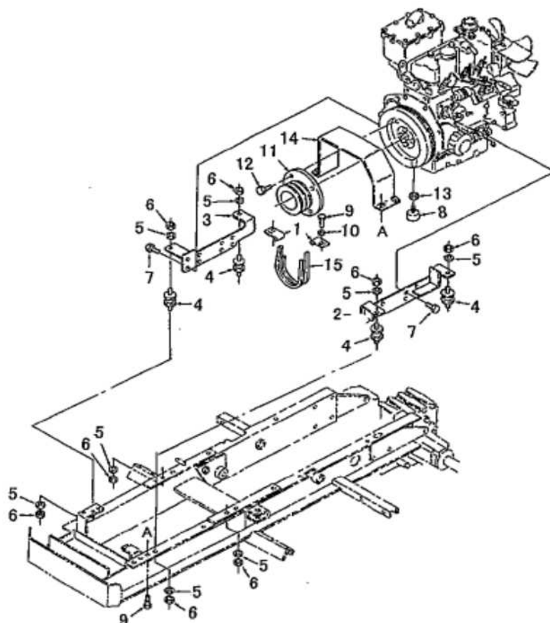
エンジンマウント ENGINE MOUNT
