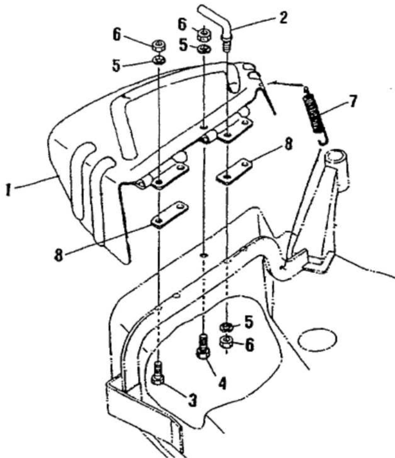
デイスチャージカバー DISCHARGE COVER
