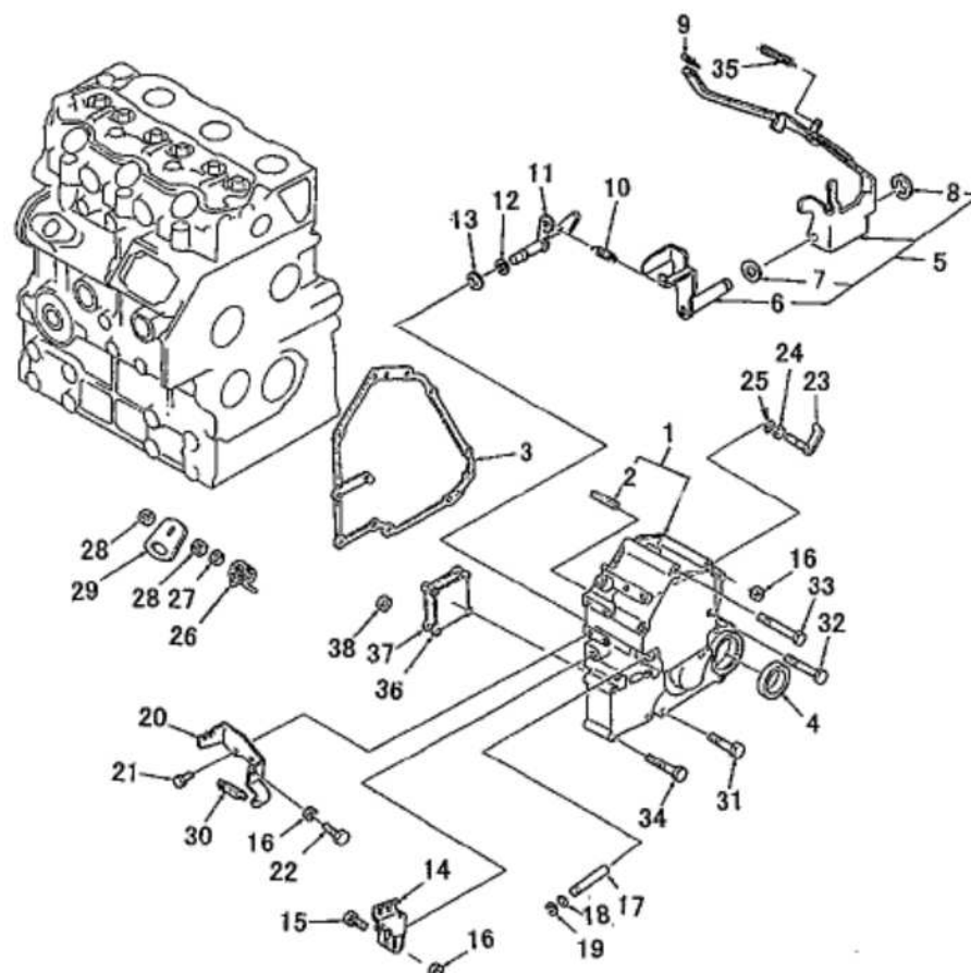
タイミングギヤケース、ガバナ TIMING GEAR CASE, GOVERNOR
