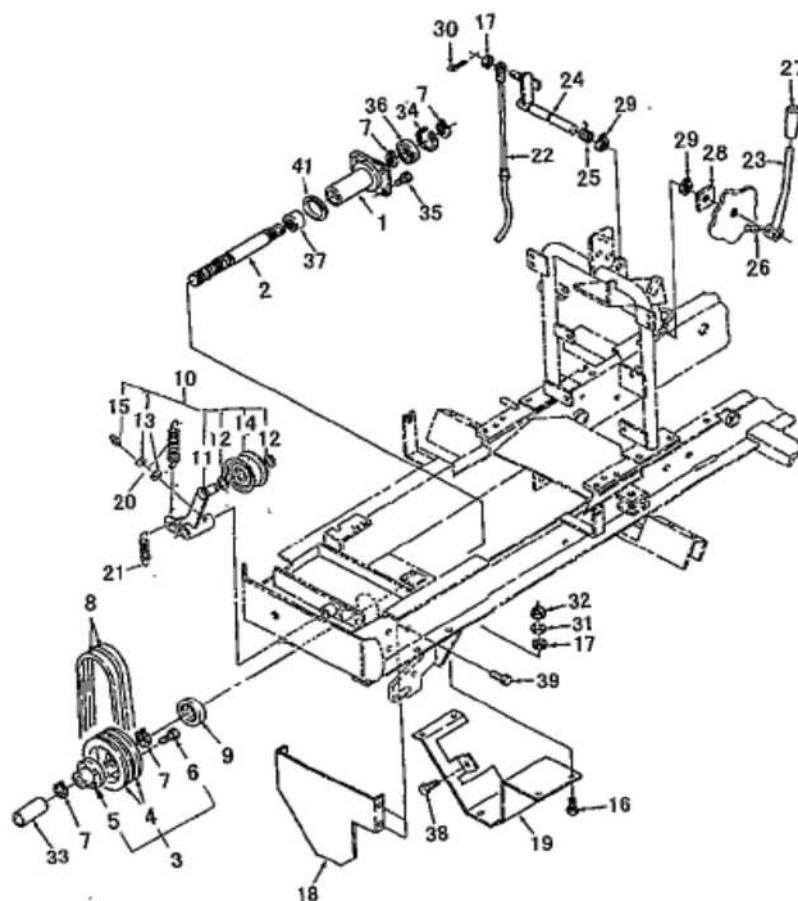
フロントPTO FRONT P.T.O
