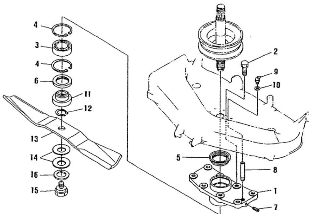
ベアリングホルダ ;センター BEARING HOLDER ;CENTER
