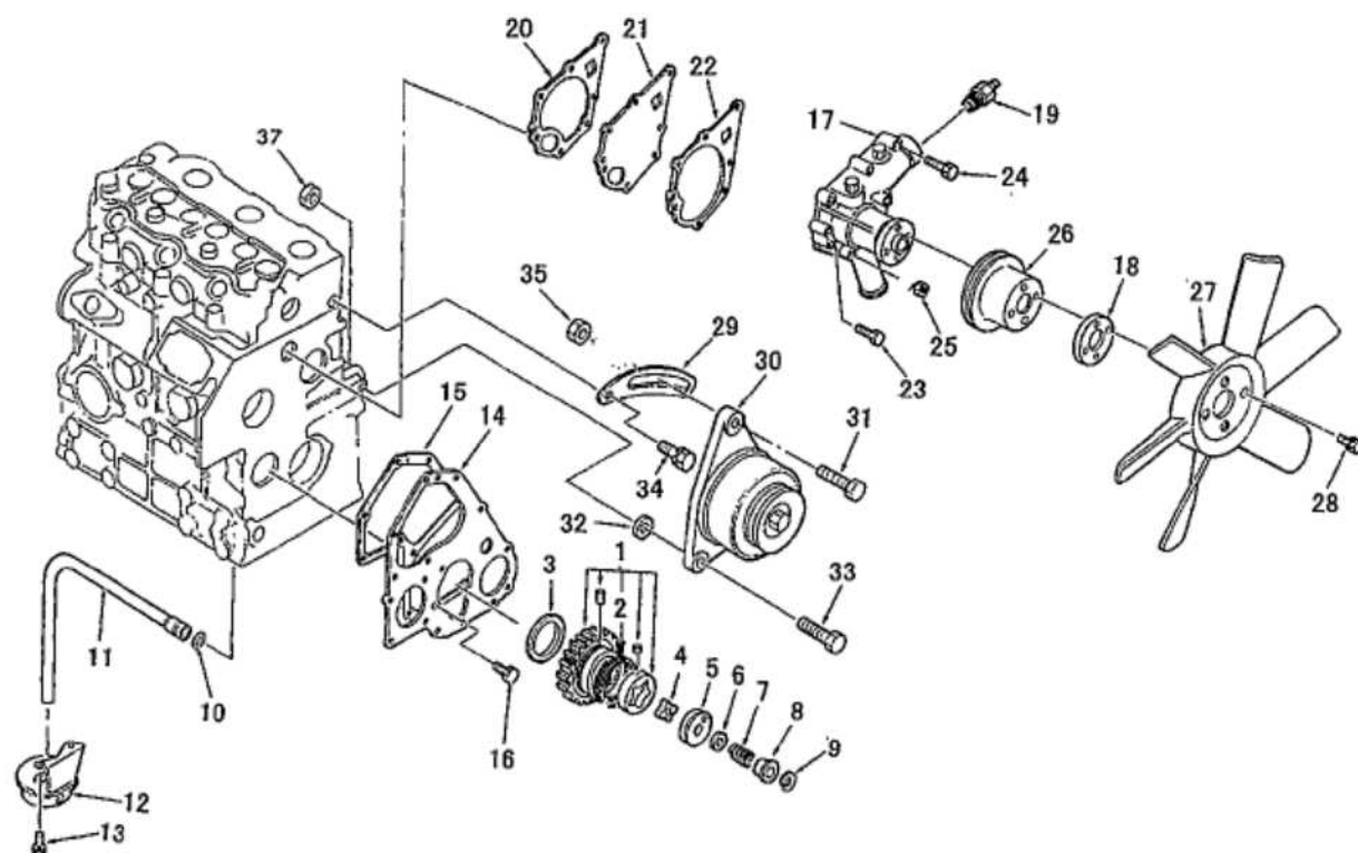
オルタネータ、ウォーターポンプ、ファン ALTERNATOR, WATER PUMP, FAN
