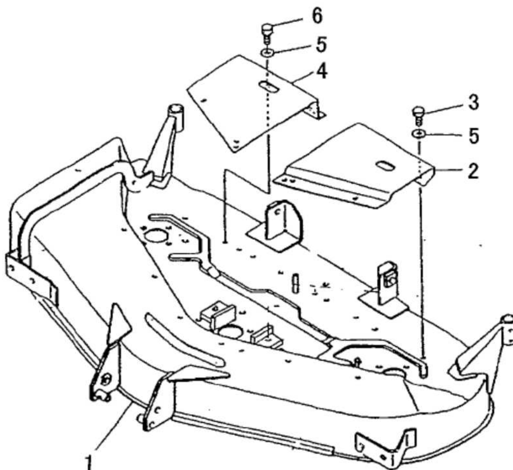
モアデツキ MOWER DECK
