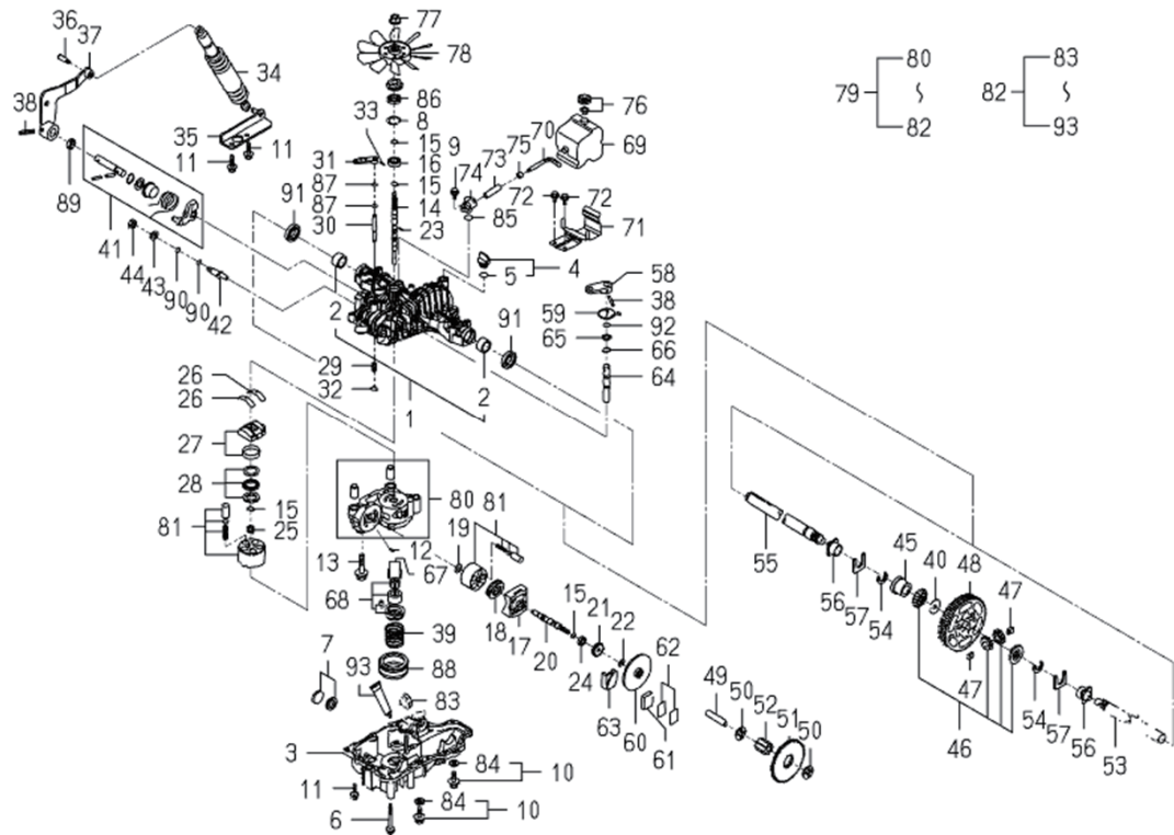
FIG.242 コンポーネントパーツ(1782-201-200-30) COMPONENT PARTS(1782-201-200-30)
