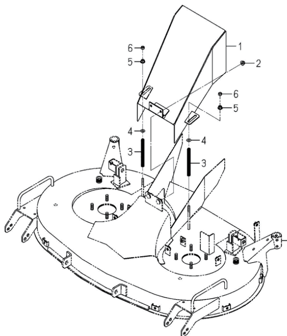
カバー COVER(DISCHARGE)SYSTEM
