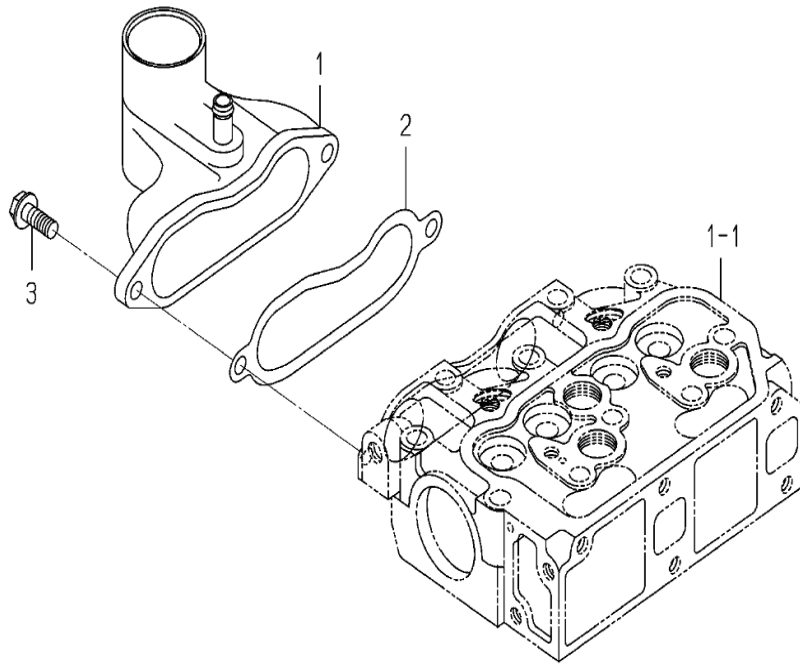
インレットマニフォールド INLET MANIFOLD
