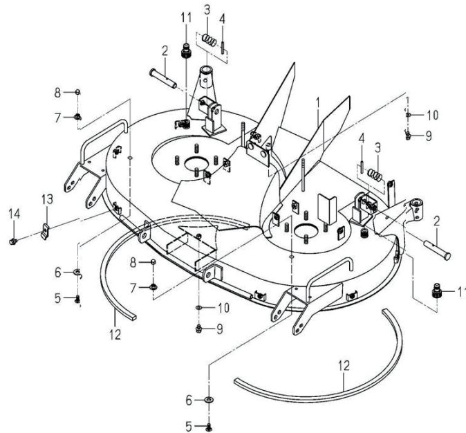
FIG.305 デッキ DECK(MOWER)SYSTEM
