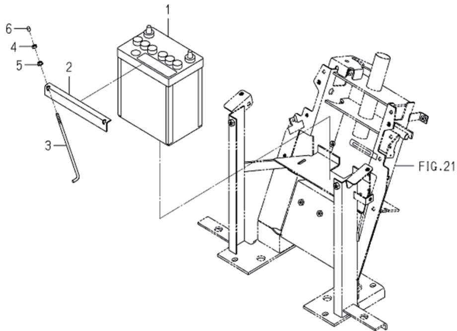
バッテリー BATTERY SYSTEM
