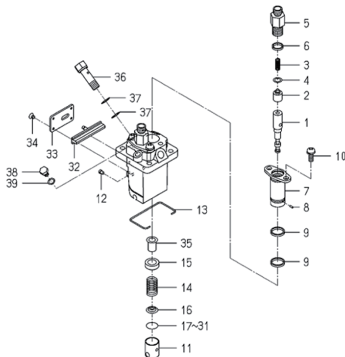
コンポーネントパーツ(6215-600-147-10) COMPONENT PARTS(6215-600-147-10)
