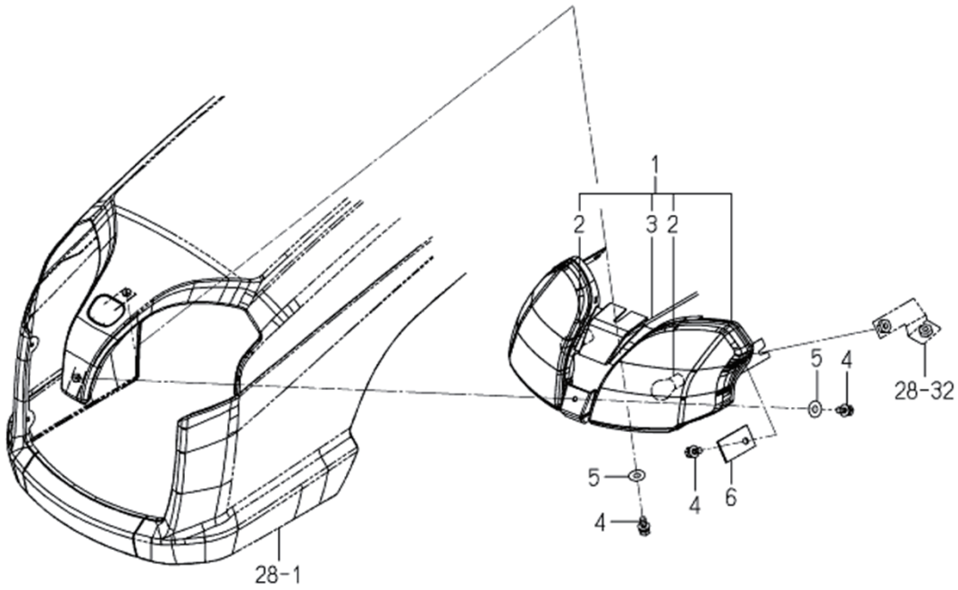
ランプ LAMP(HEAD)SYSTEM
