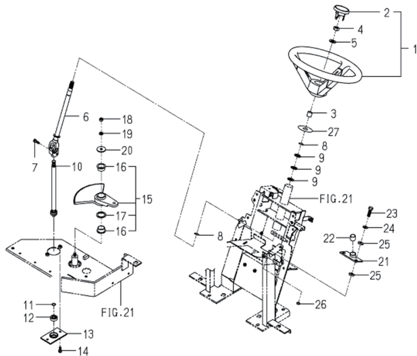
シャフト FIG.220 SHAFT(STEERING)SYSTE M
