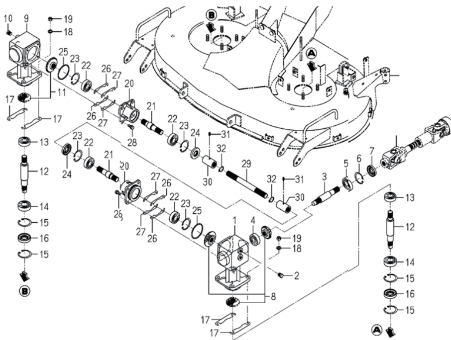
ケース(ベベル) CASE(BEVEL)SYSTEM
