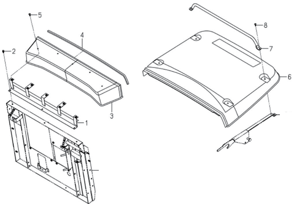
カバー(コンテナ) COVER(CONTAINER)SYSTEM
