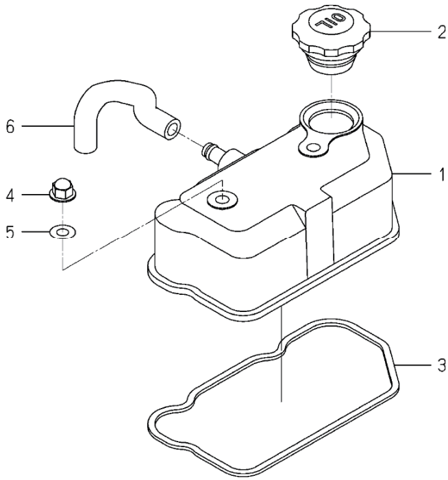
シリンダーヘッドカバー CYLINDER HEAD COVER
