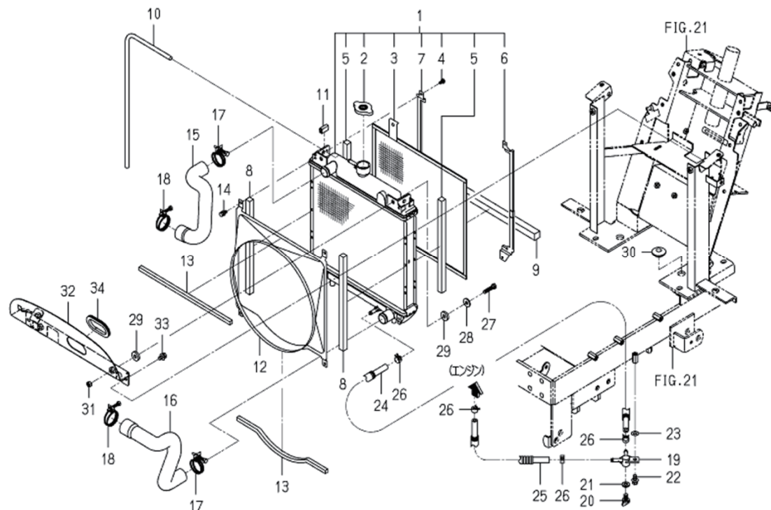
FIG.202 ラジエータ RADIATOR SYSTEM
