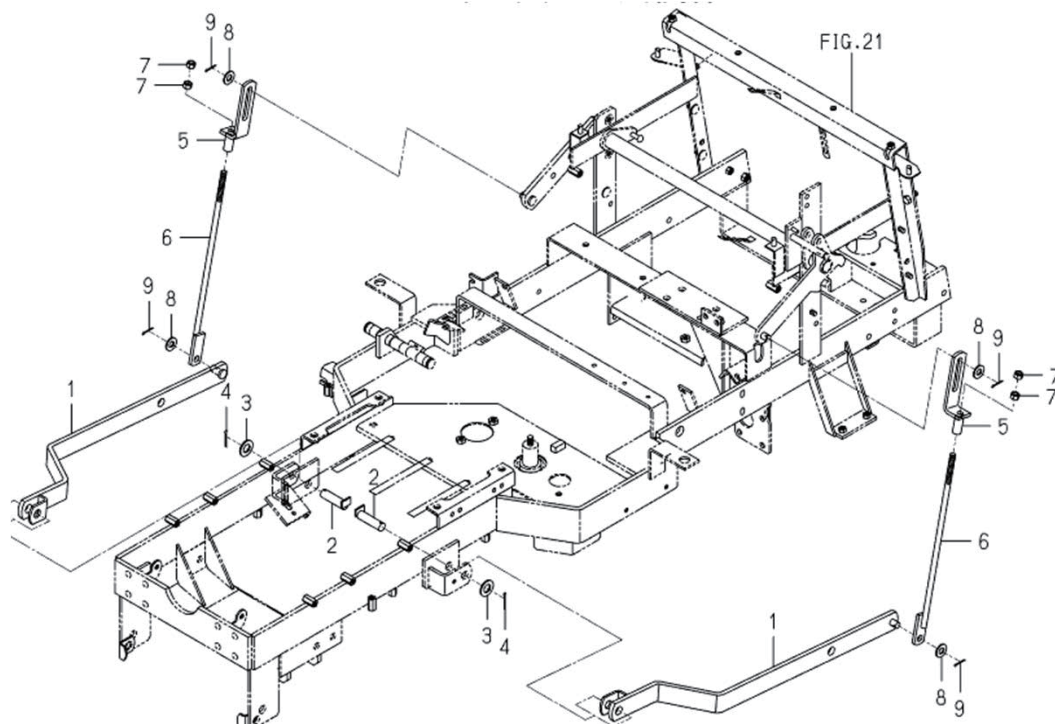
リンク LINK(MOWER)SYSTEM
