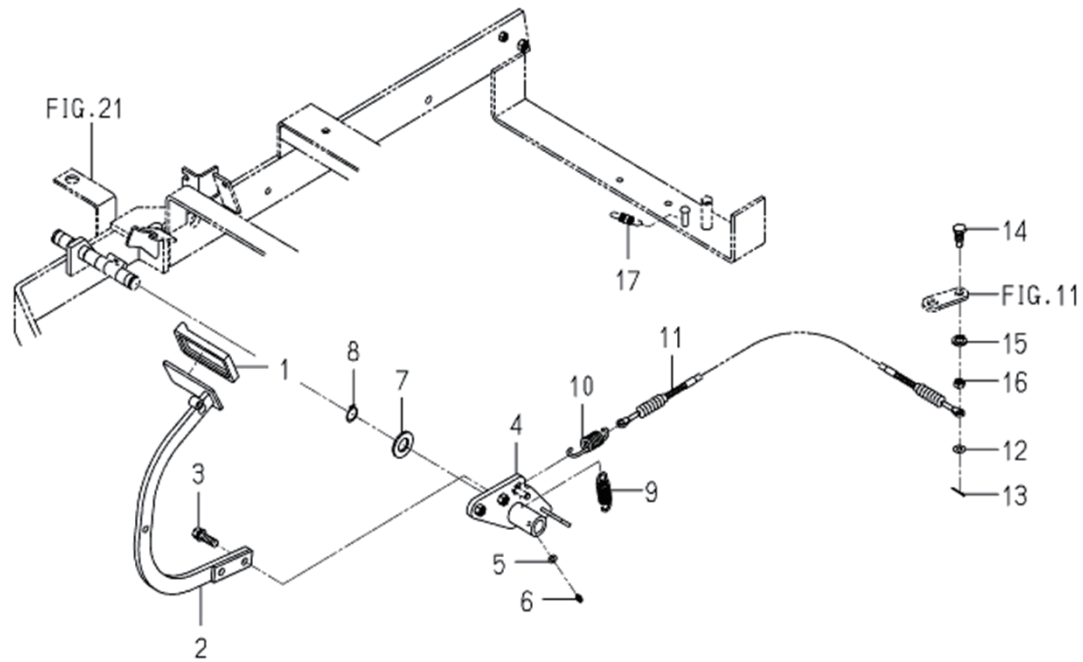
FIG.216 ペダル PEDAL(BRAKE)SYSTEM
