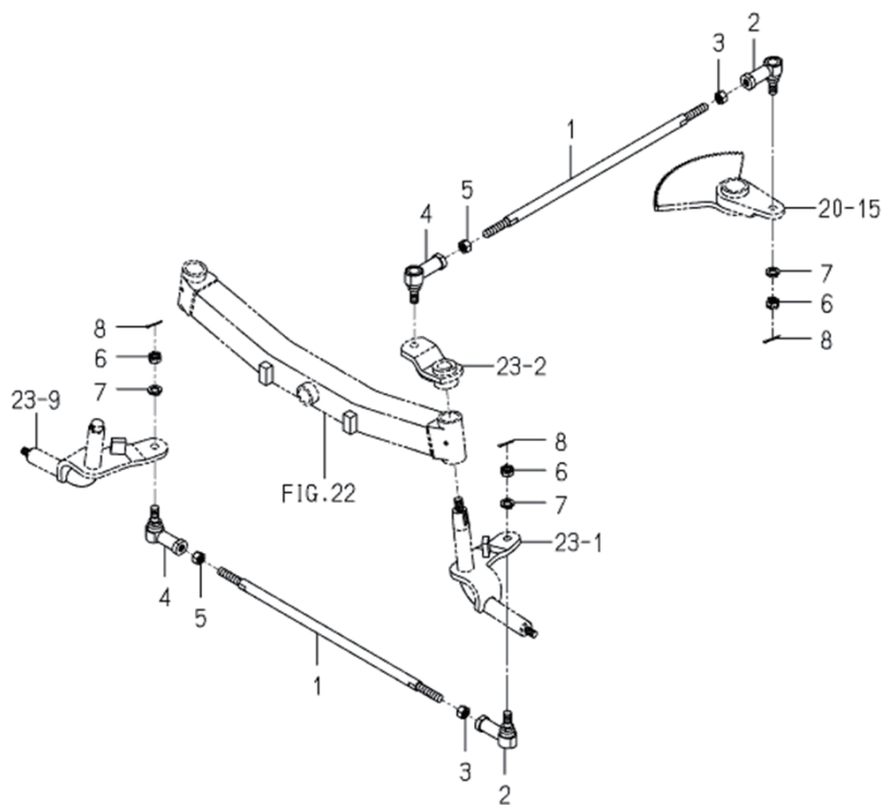
ロッド ROD(TIE)SYSTEM
