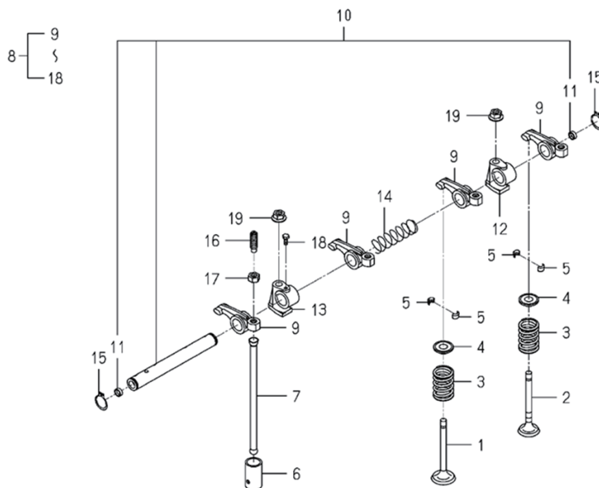
FIG.112 バルブ VALVE
