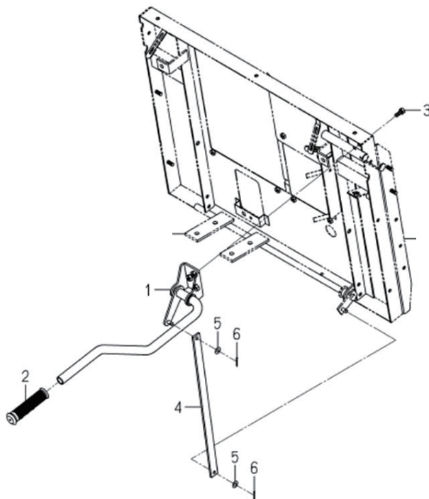
レバー LEVER(CLEANER)SYSTEM
