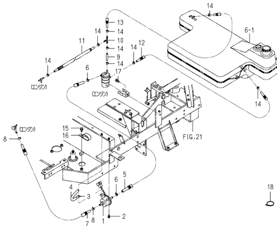
FIG.205 ポンプ PUMP(FUEL)SYSTEM
