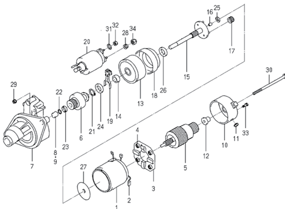
コンポーネントパーツ(6281-100-014-00) COMPONENT PARTS(6281-100-014-00)
