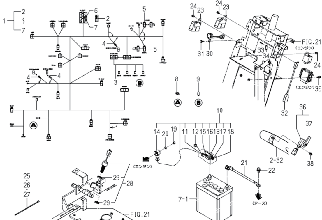
FIG.236 ハーネス HARNESS SYSTEM
