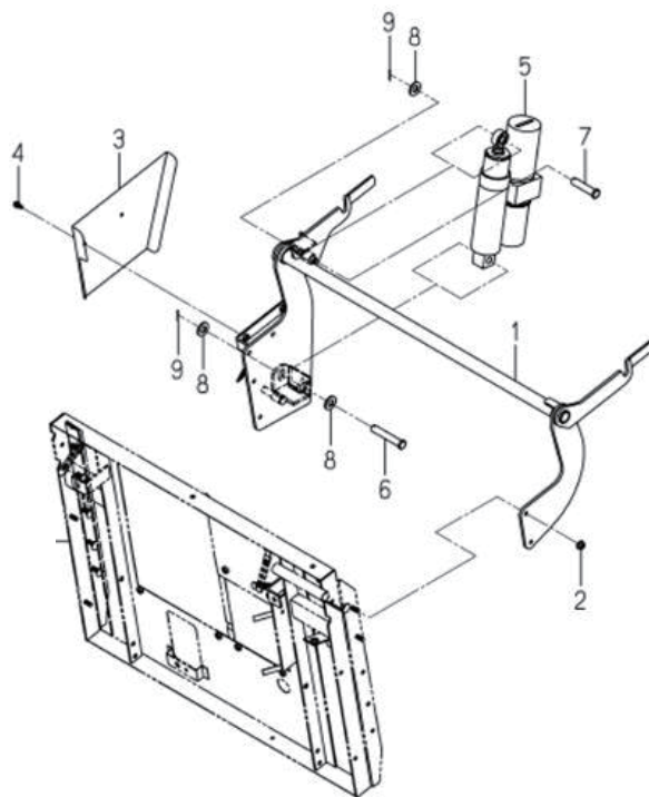
リフト LIFT SYSTEM(A TYPE)
