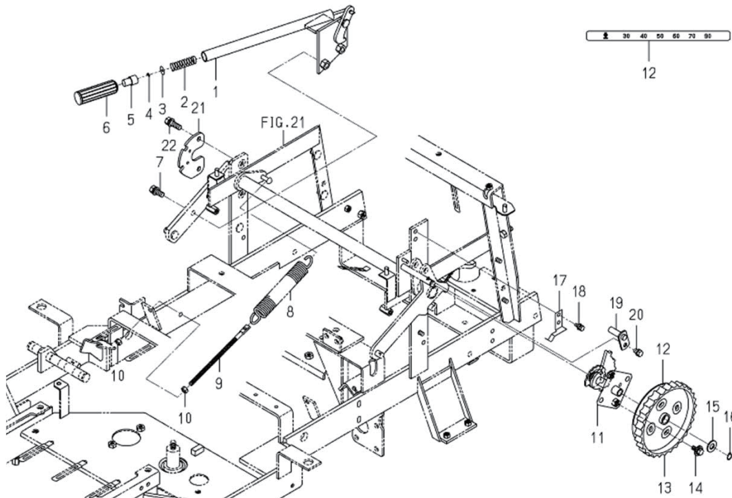
FIG.227 レバー(リフト) LEVER(LIFT)SYSTEM
