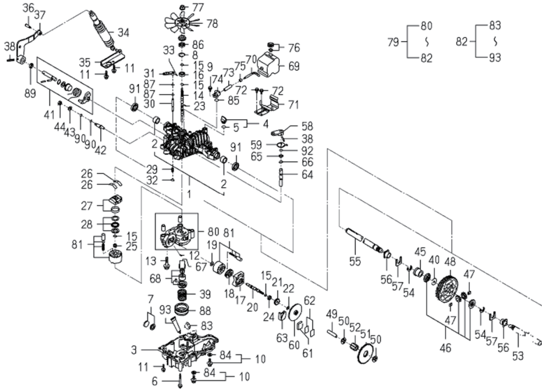
コンポーネントパーツ(1782-201-200-30) COMPONENT PARTS(1782-201-200-30)
