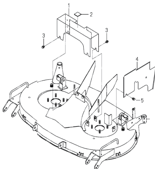
カバー COVER SYSTEM
