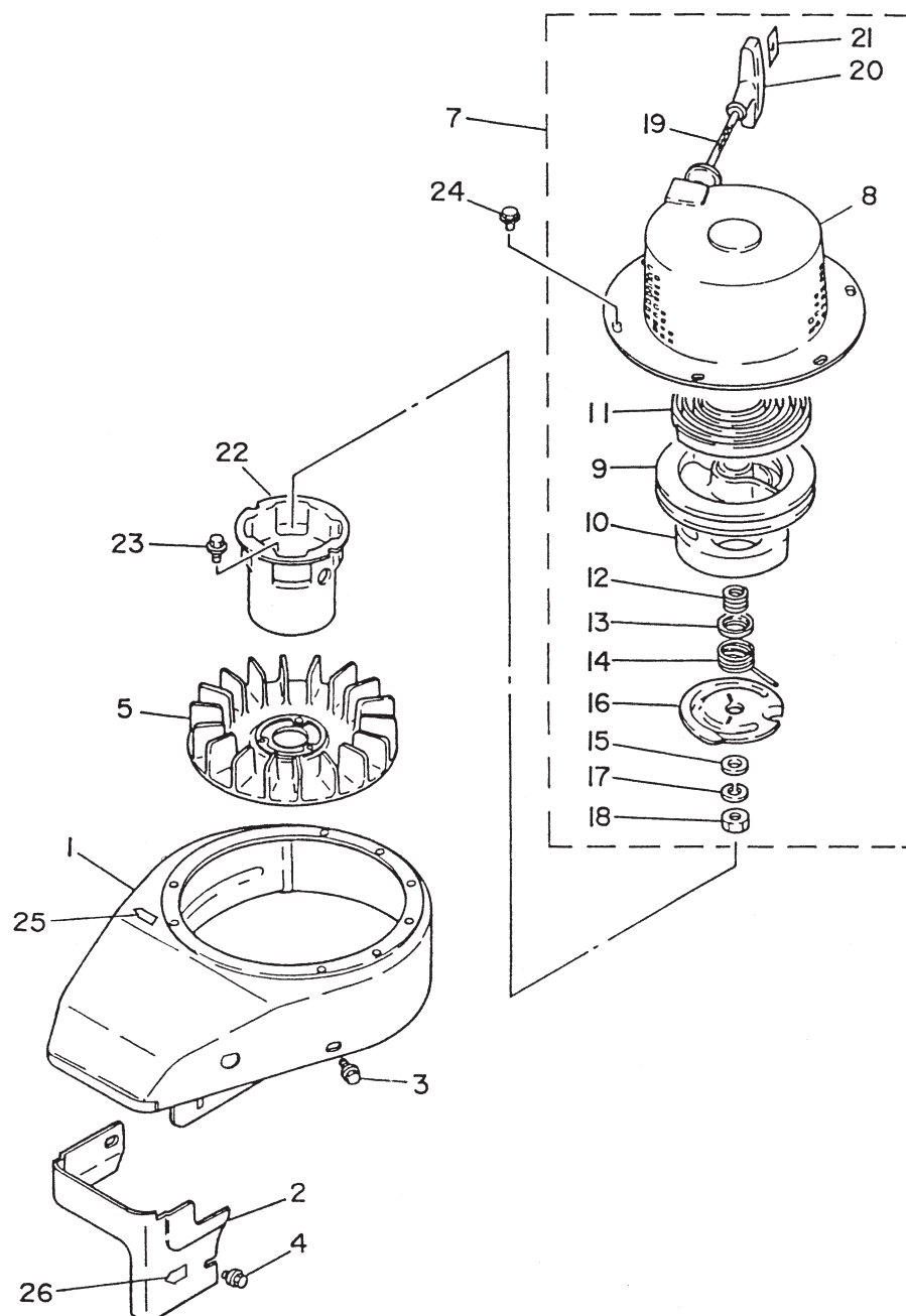
第4図 エアシュラウド・スタータ
