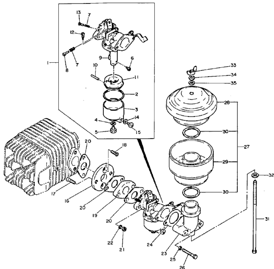
第4図 インテーク・キャブレタ
