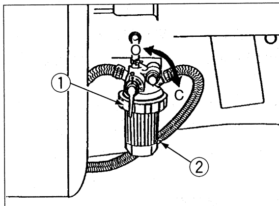
①燃料コック ②フィルタカップ
