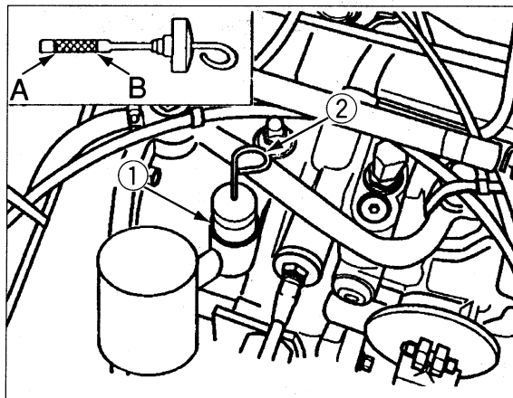
1. 給油口 A. 下限 2. 検油ゲージ B. 上限
