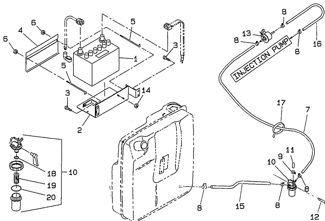
FIG.201 フュエルライン, バッテリ FUEL LINES, BATTERY
