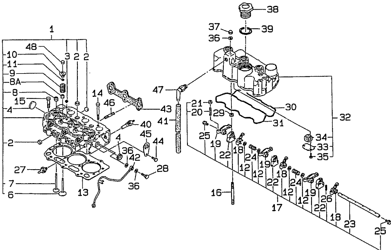
シリンダヘッド FIG.103 CYLINDER HEAD ; MC234
