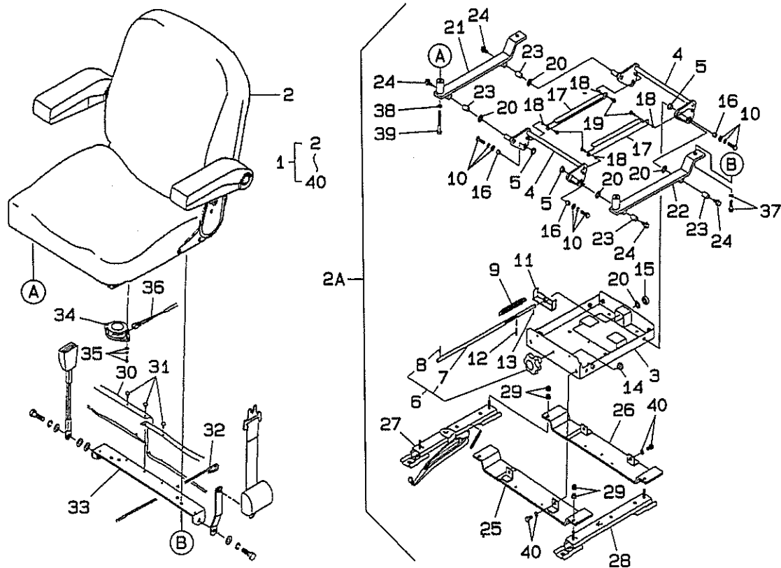
シート FIG.223A SEAT
