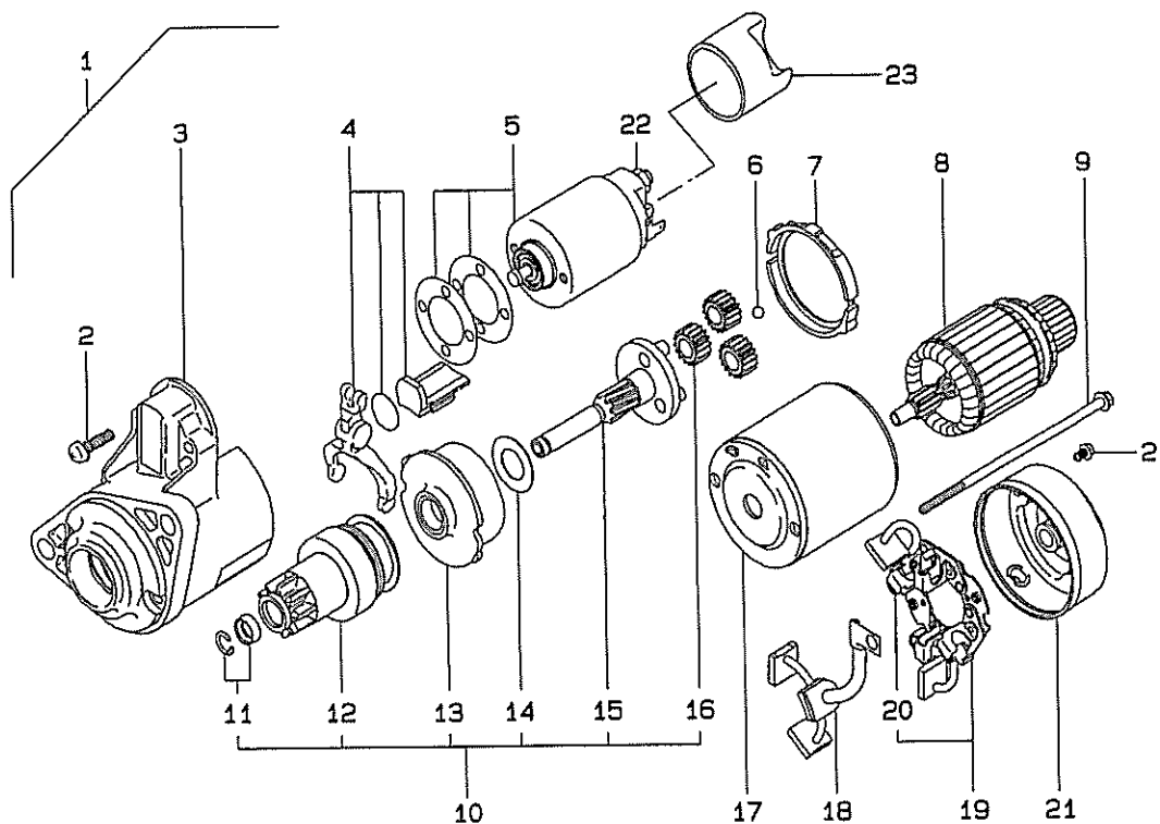
FIG.118 スターティングモータ STARTING MOTOR ; MC284
