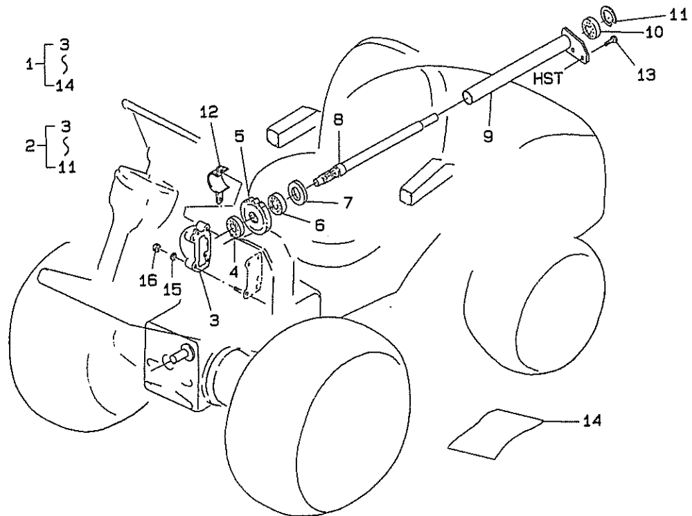
FIG.233 サイド P.T.O SIDE P.T.O
