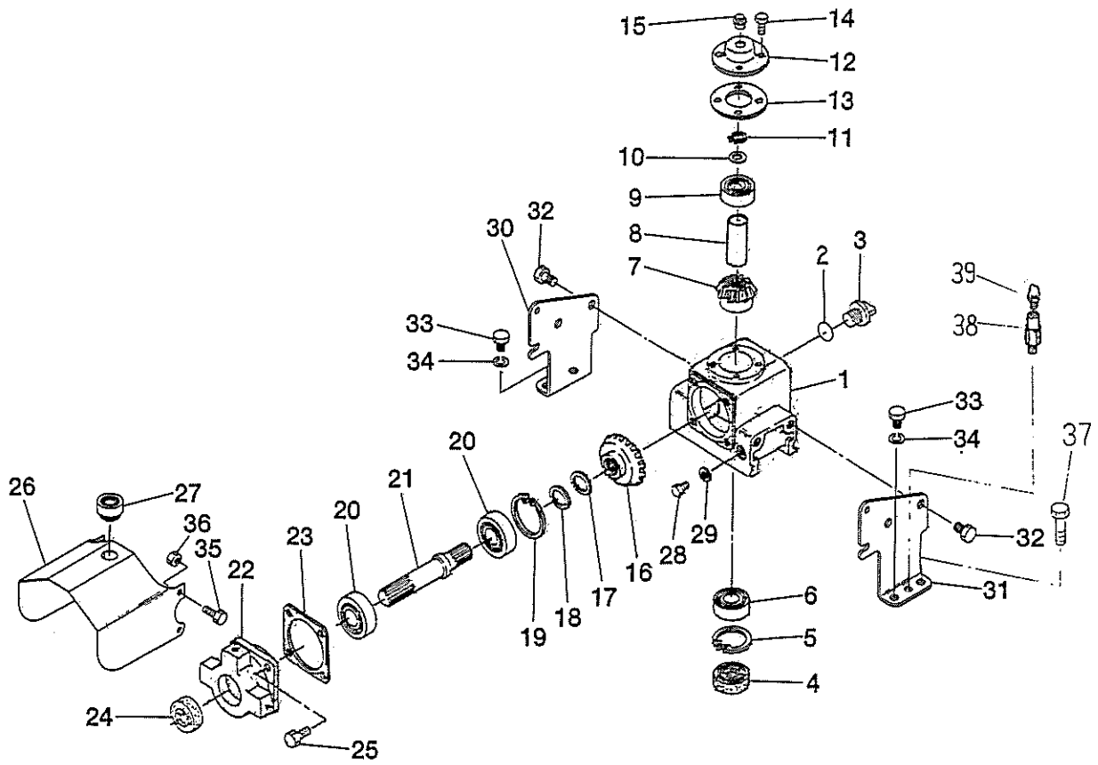
ギヤボックス GEAR BOX
