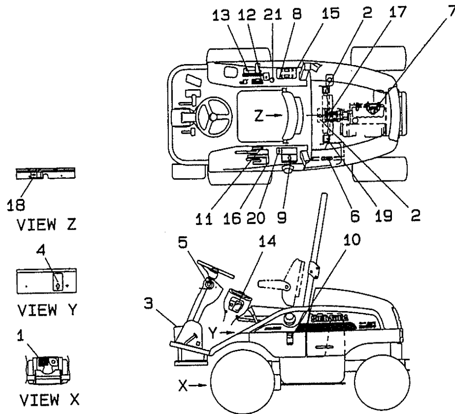
FIG.232 コーシヨンプレート CAUTION PLATE
