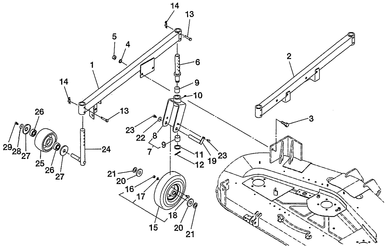
ゲージホイール FIG.305 GAUGE WHEELS
