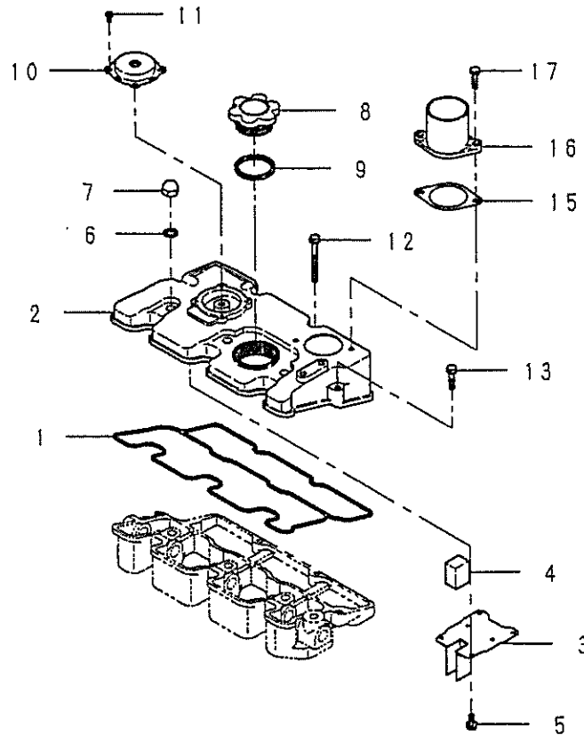
FIG.104B ヘッドカバー；ティアⅡ ☆ HEAD COVER； MC284/MC354
