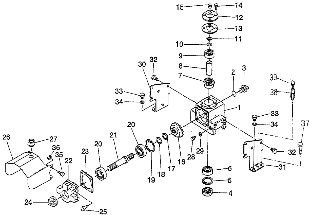
ギヤボックス FIG.302 GEAR BOX
