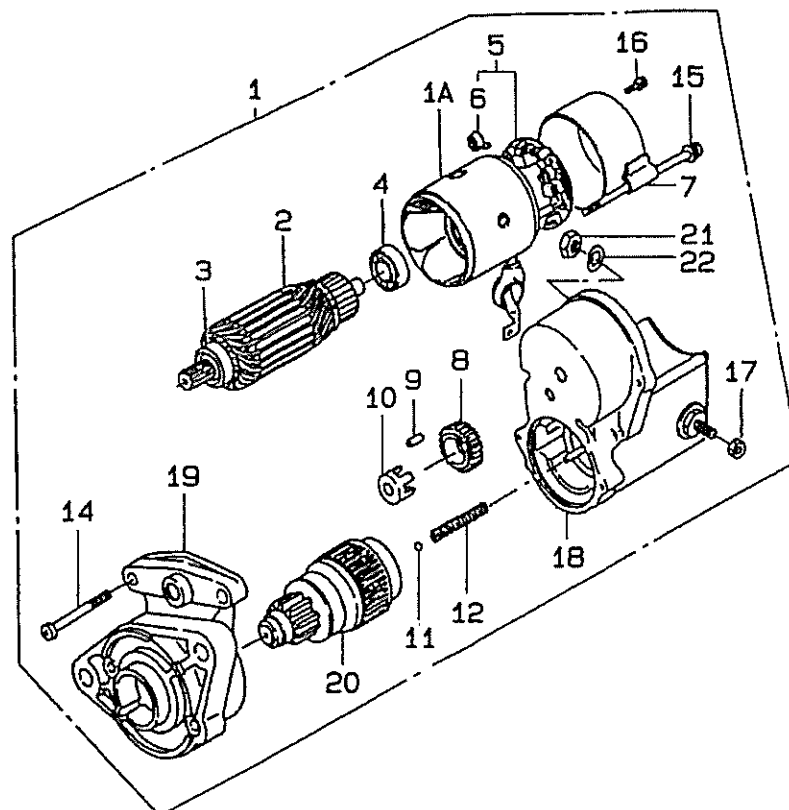
FIG.117 スターティングモータ STARTING MOTOR ; MC234
