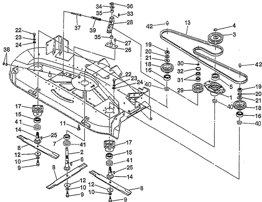
FIG.303 プーリ, ブレード PULLEY, BLADE
