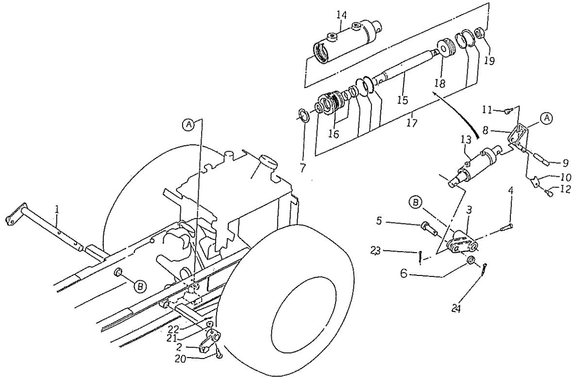
FIG.218 リフトシリンダ LIFT CYLINDER
