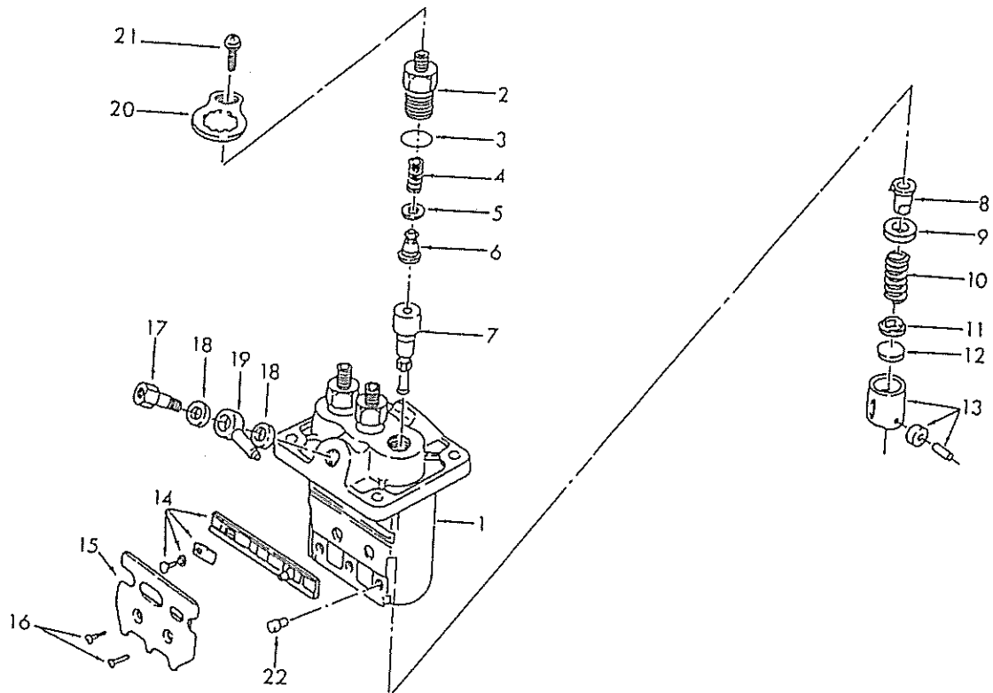
FIG.108 インジェクションポンプ INJECTION PUMP
