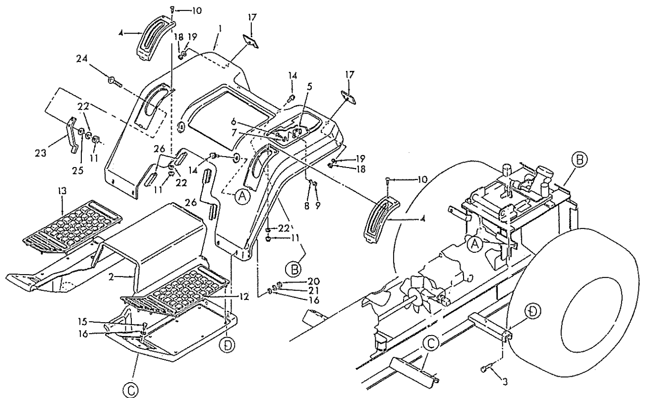
FIG.227 ステップ, フェンダ STEPS, FENDERS
