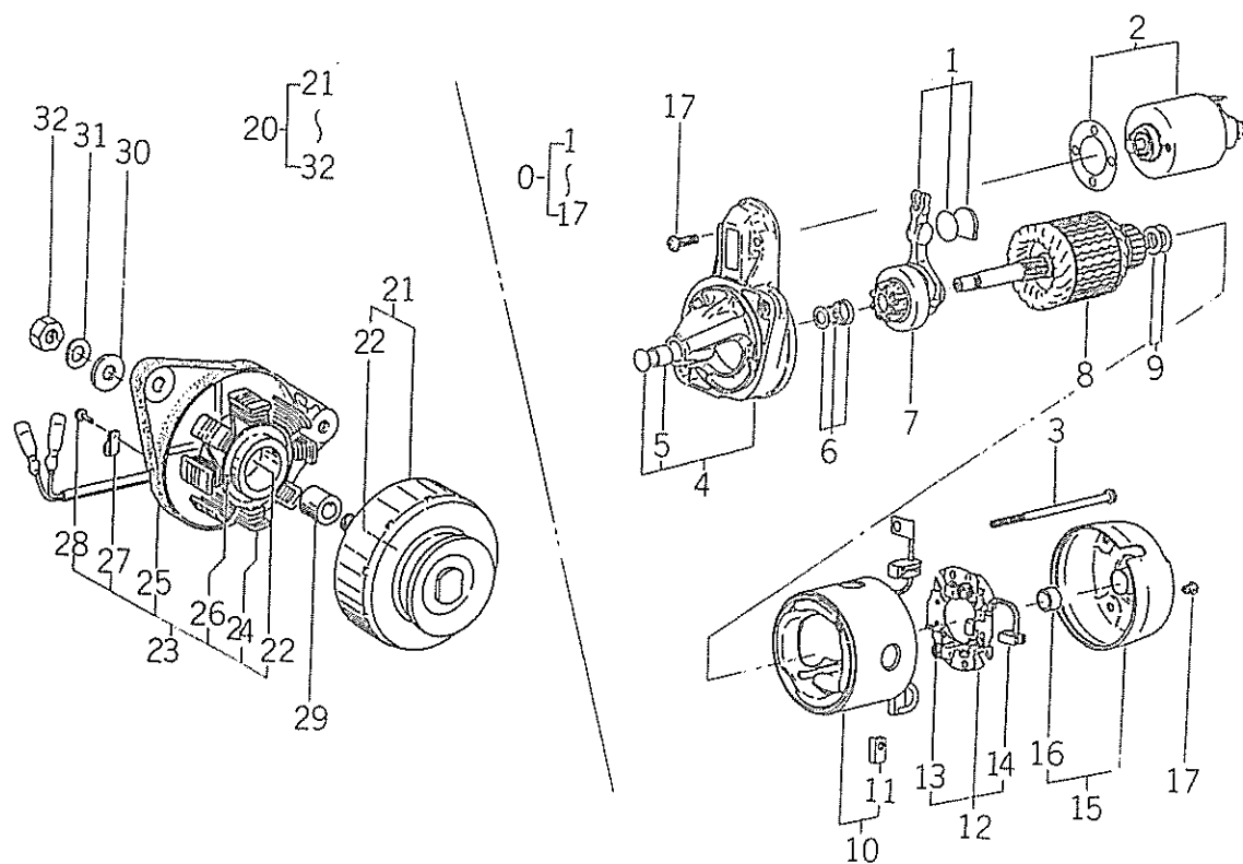
FIG.112 スタータ, オルタネータ STARTER, ALTERNATOR
