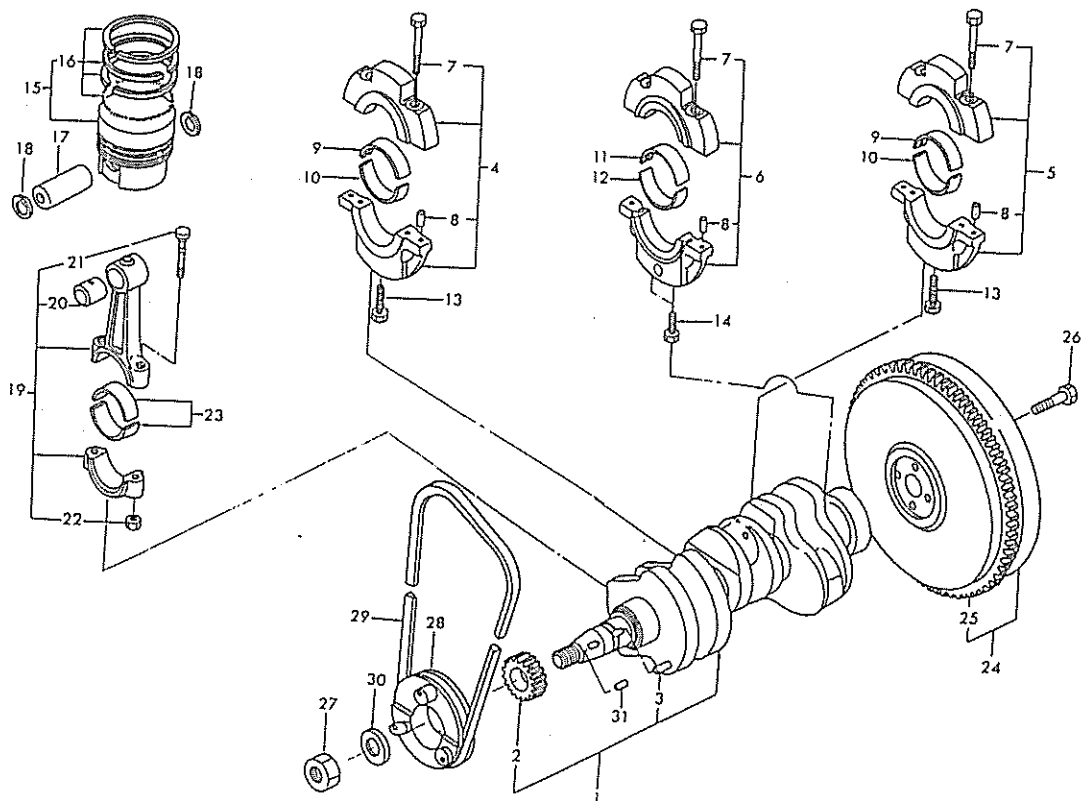
クランクシャフト, ピストン CRANKSHAFT, PISTON
