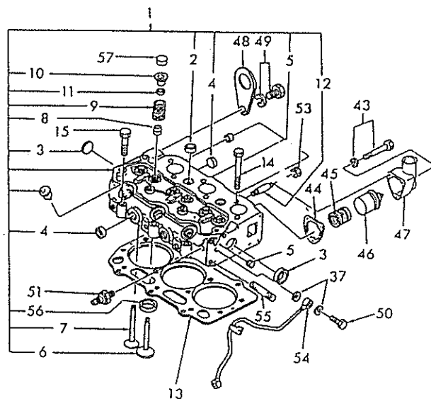
FIG.103 シリンダヘッド CYLINDER HEAD
