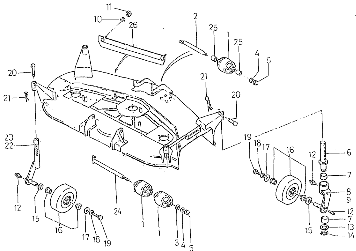
FIG.315 ゲージホイール, ローラ GAUGE, WHEEL, ROLLER ; 60"
