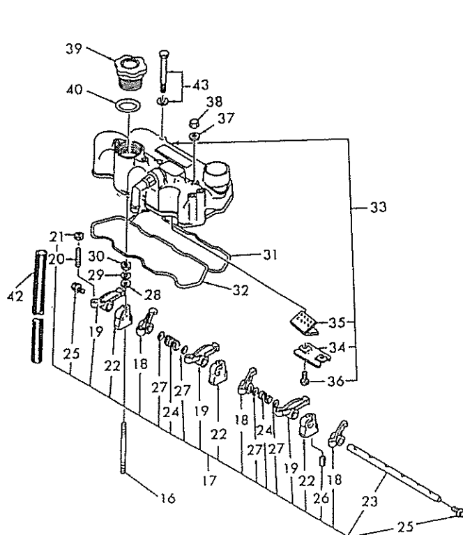
FIG.103 シリンダヘッド CYLINDER HEAD
