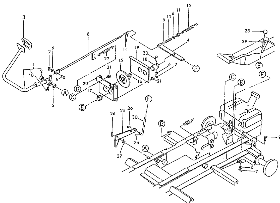
FIG.214 ブレーキ BRAKE
