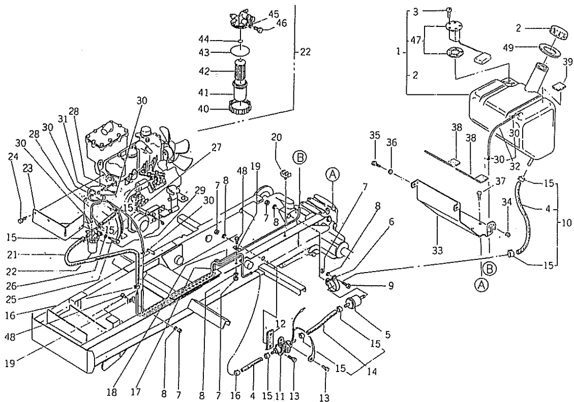
FIG.219 フューエルライン FUEL LINE ; DIESEL
