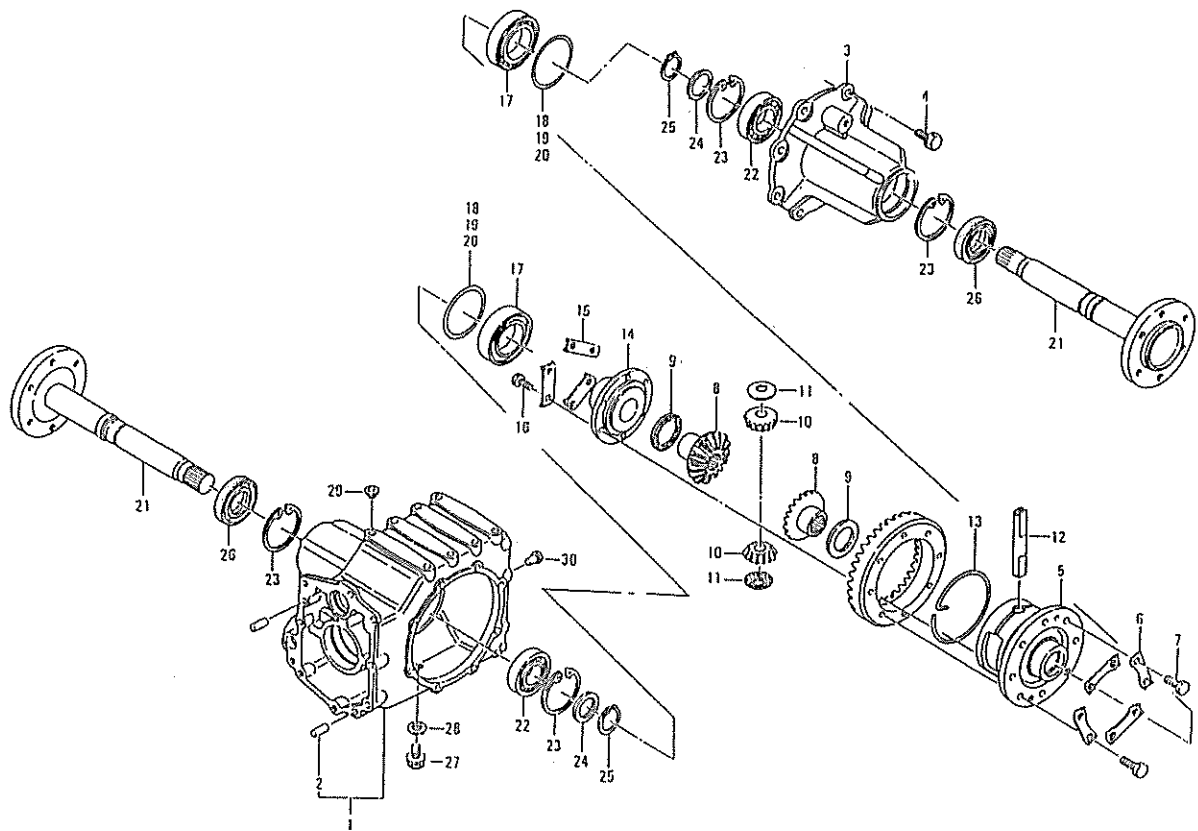
FIG.212 ホイルシャフトケース WHEEL SHAFT CASE
