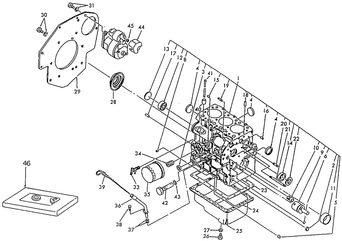
シリンダブロック CYLINDER BLOCK
