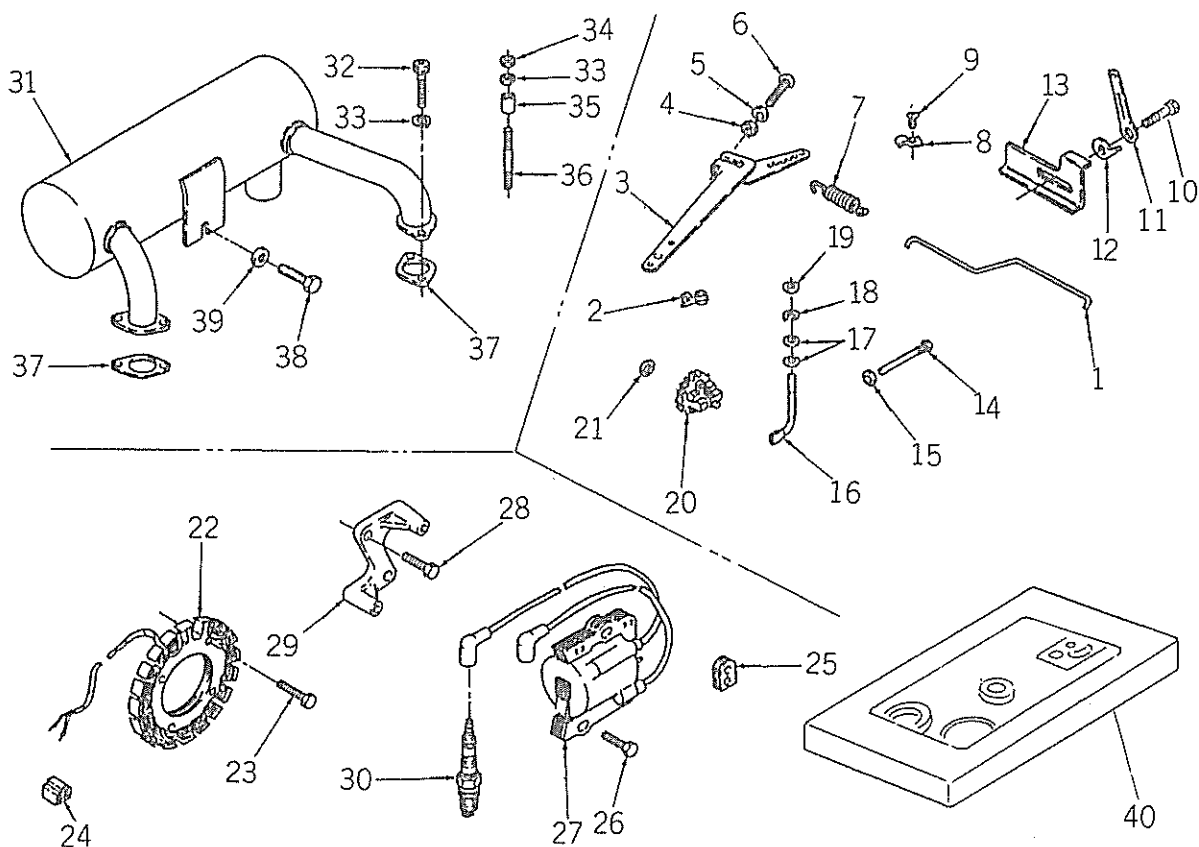
FIG.126 ガバナ, イグニション, マフラ, ガスケットセット GOVERNOR, IGNITION, MUFFLER, GASKET SET
