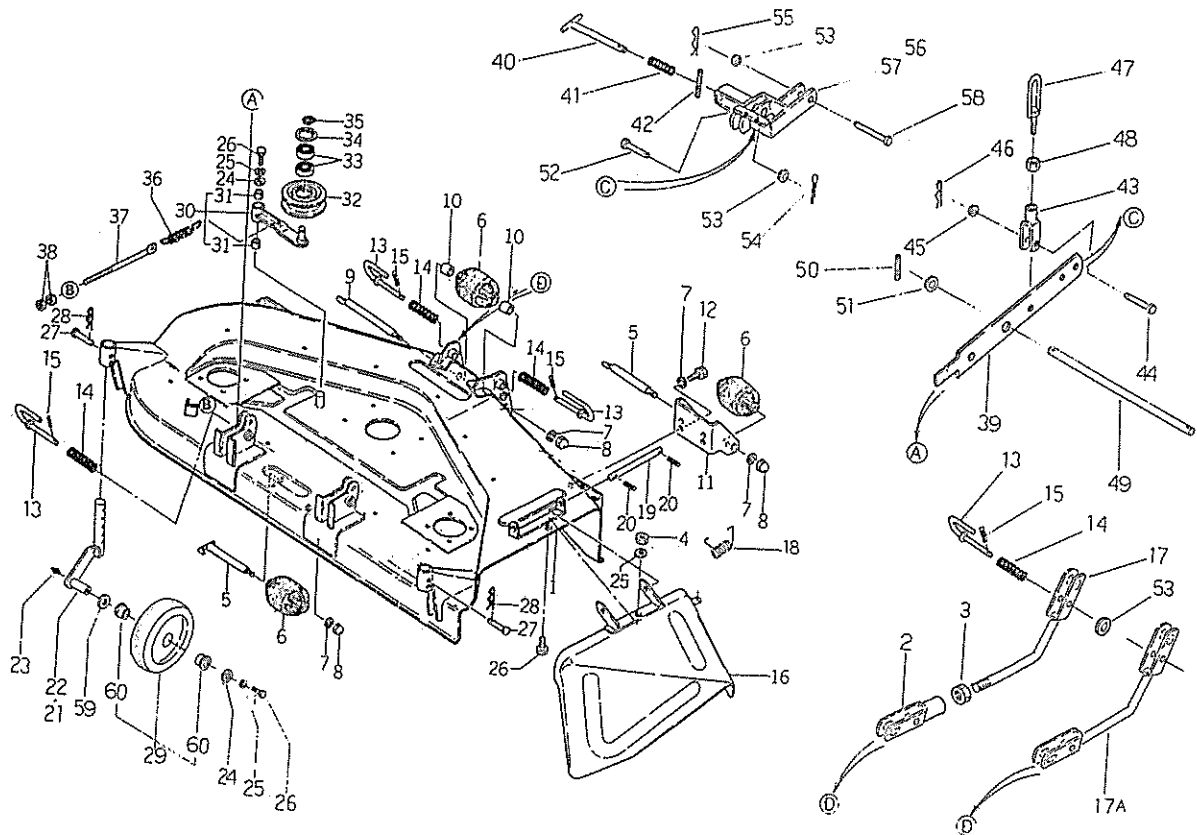
FIG.302 モアデッキ, リンク MOWER DECK, LINK ; 44" & 48"
