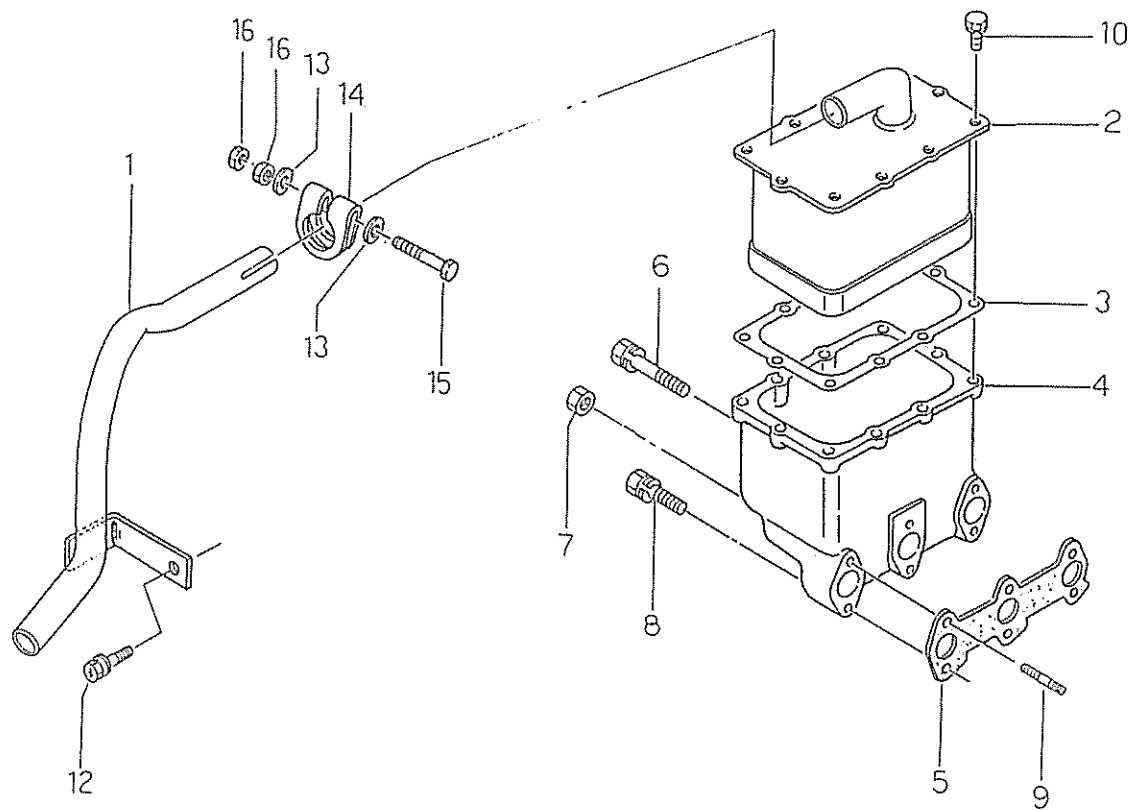
FIG.111 マフラ MUFFLER
