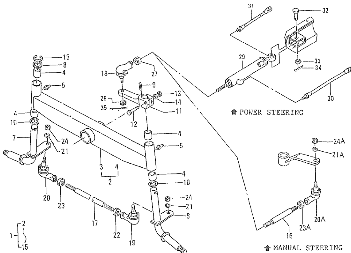
FIG.202 フロントアクスル FRONT AXLE
