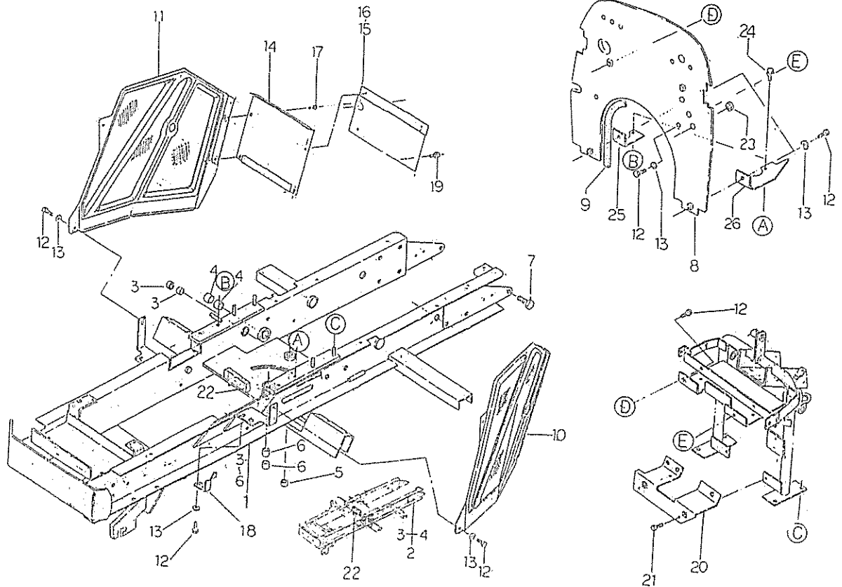
FIG.208 シャーシ、ダッシュボード CHASSIS, DASH BOARD ; GASOLINE
