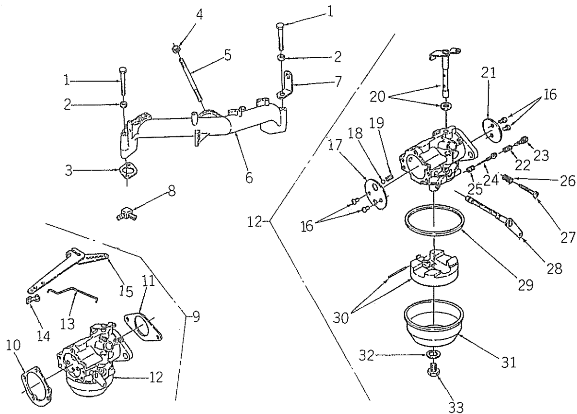
FIG.123 マニホルド, キャブレータ MANIFOLD, CARBURETOR
