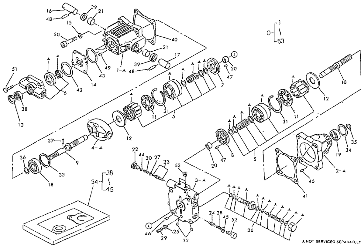
FIG.210 油圧モータ ; H. S. T HYDRO STATIC TRANSMISSION
