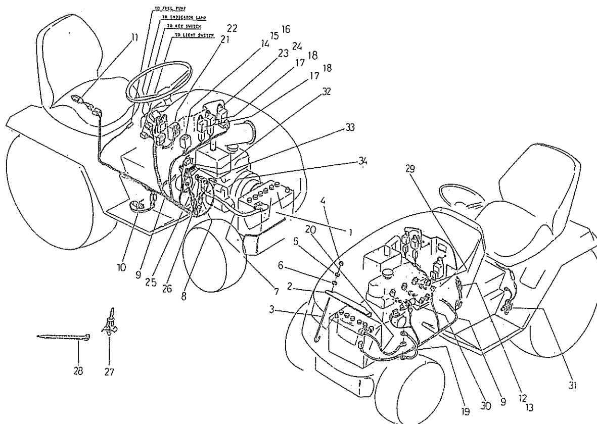
FIG.222 配線系統 WIRING HARNEES ; DIESEL
