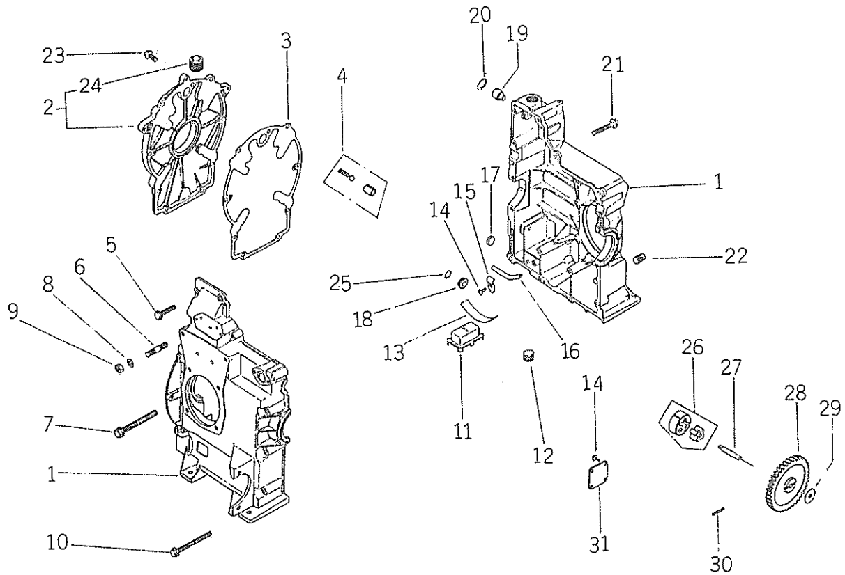
FIG.121 クランクケース CRANK CASE
