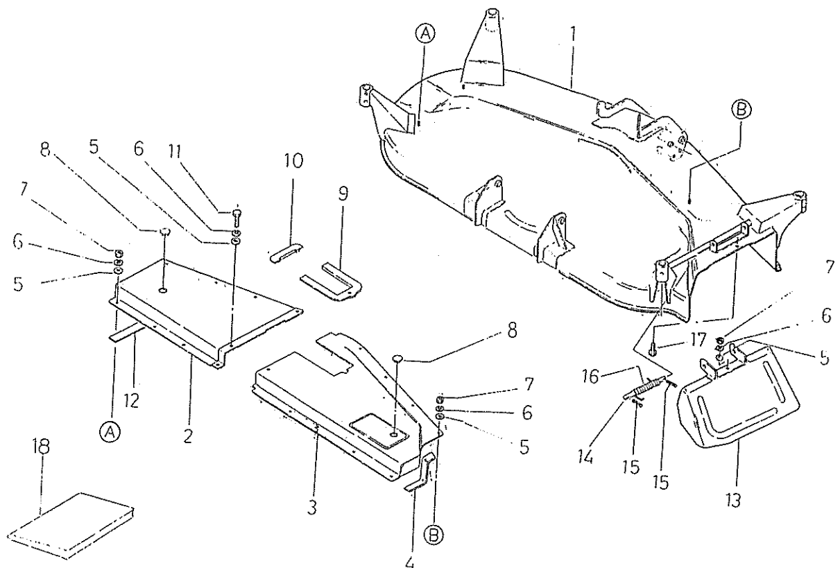
FIG.313 モアデッキ, カバー MOWER DECK, COVER ; 60"
