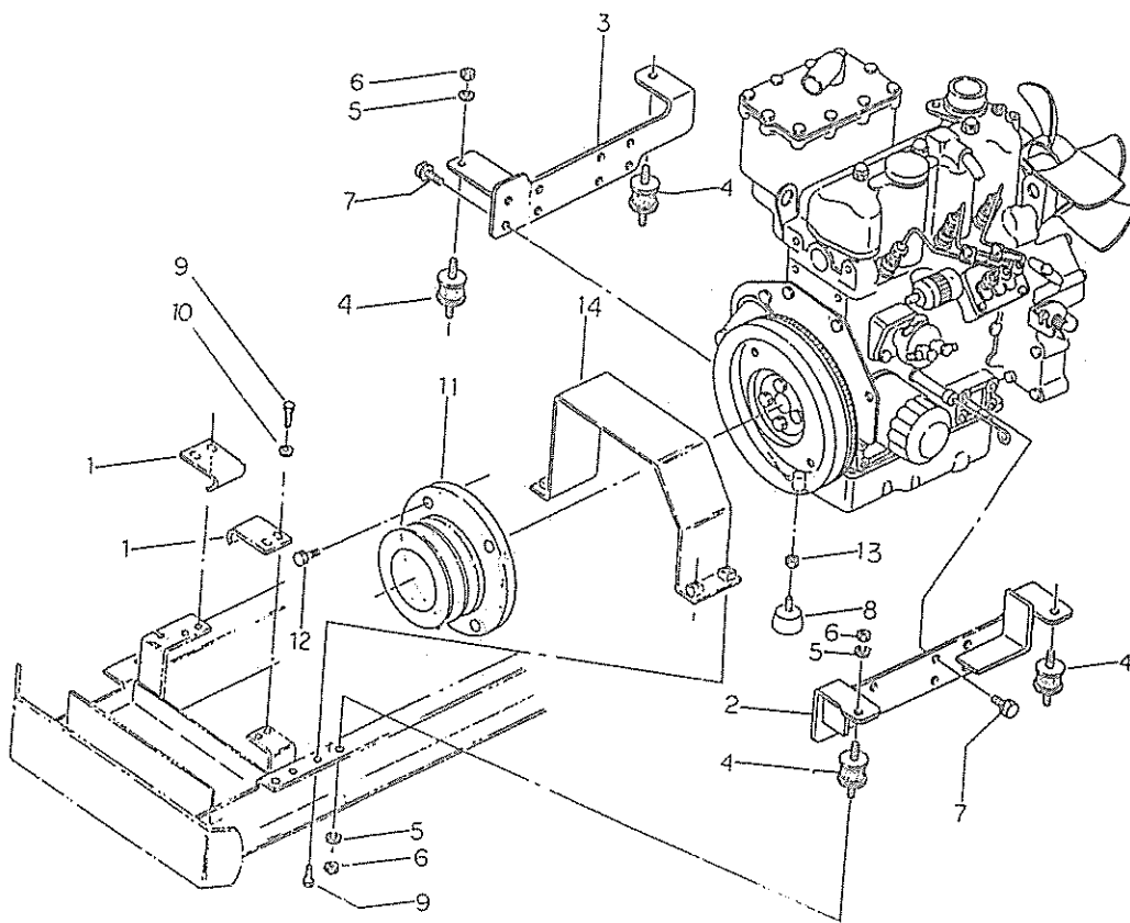
エンジンマウント ENGINE MOUNT
