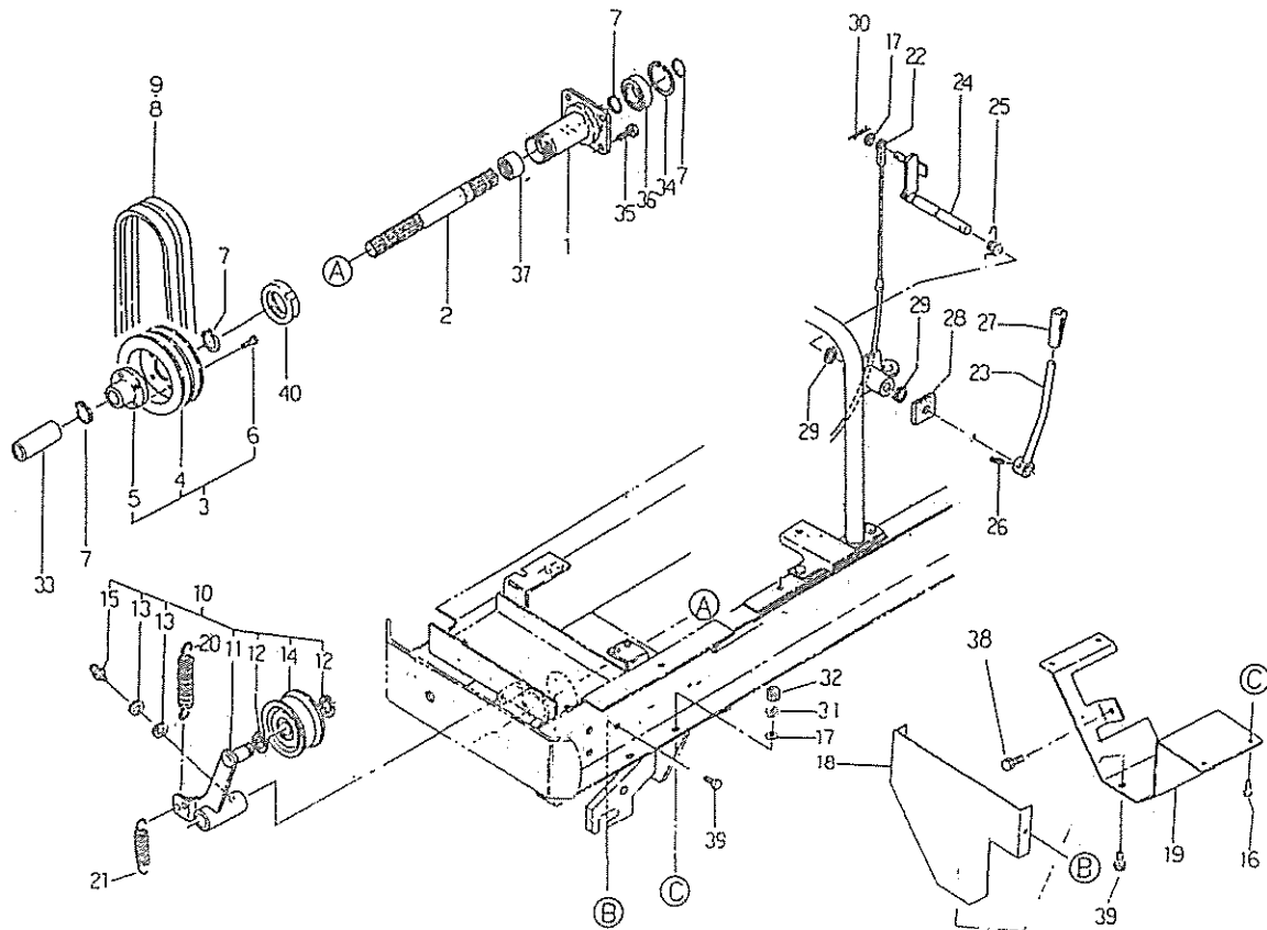
フロント P. T. 0 FRONT P. T. 0
