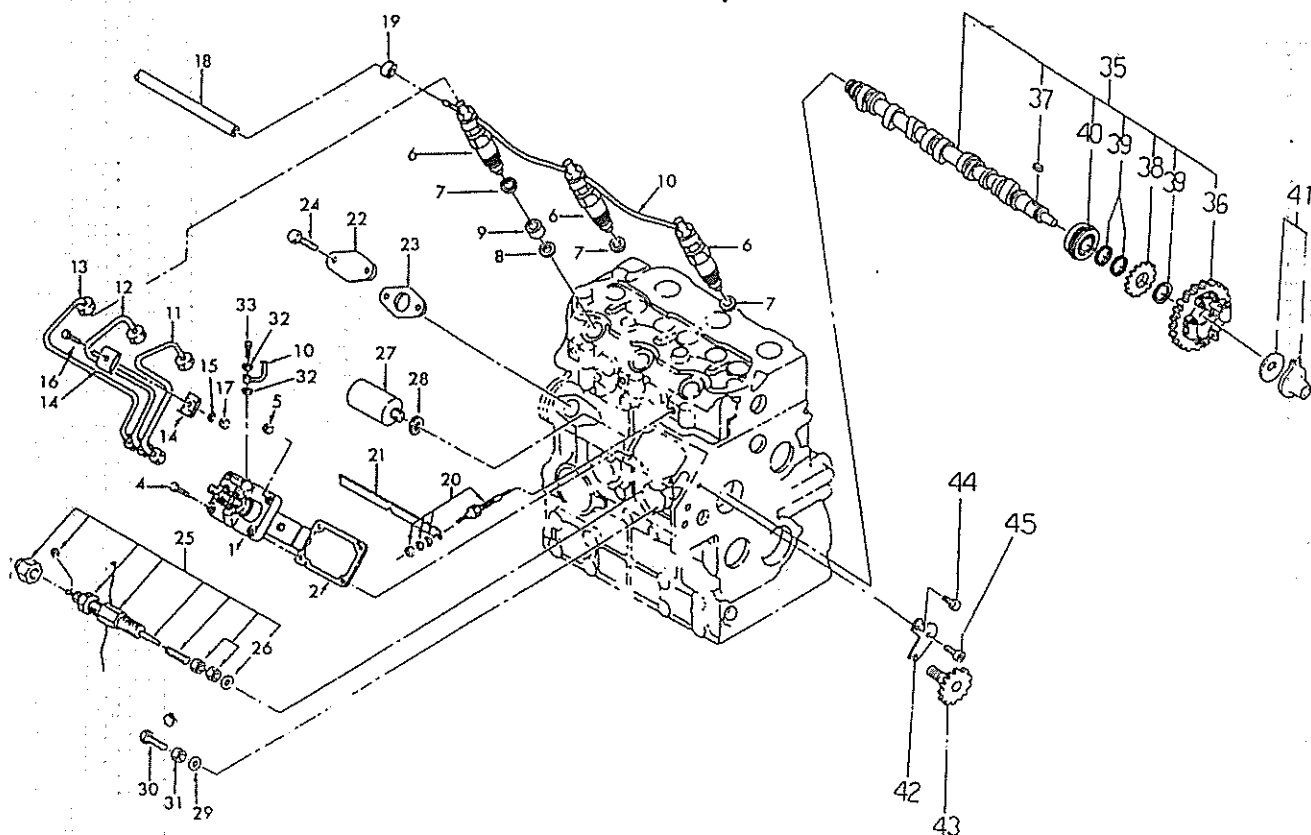
FIG.107 インジェクションライン, カムシャフト INJECTION LINE, CAMSHAFT
