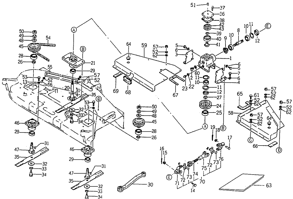
FIG.301 ギヤボックス, ブレード GEAR BOX, BLADE ; 44 "&48"
