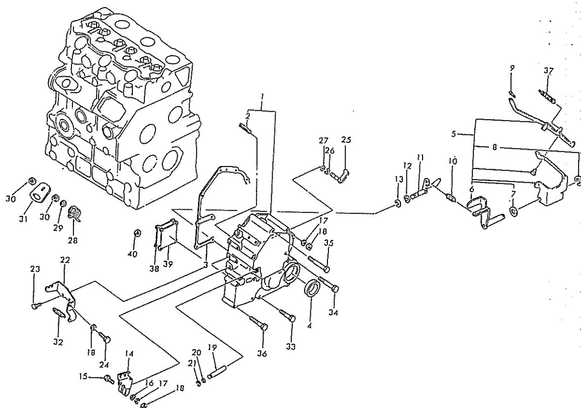
FIG.106 タイミングギヤケース TIMING GEAR CASE
