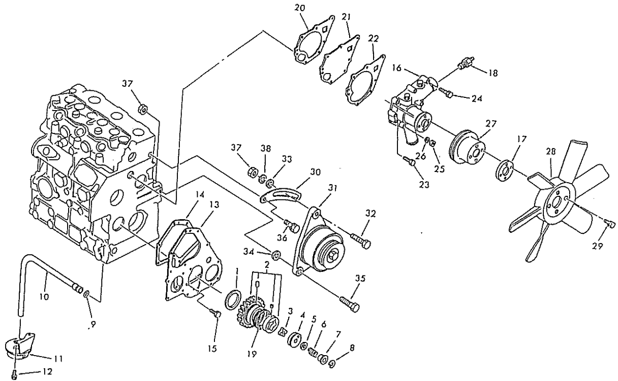
オイルポンプ, ウォーターポンプ OIL PUMP, WATER PUMP
