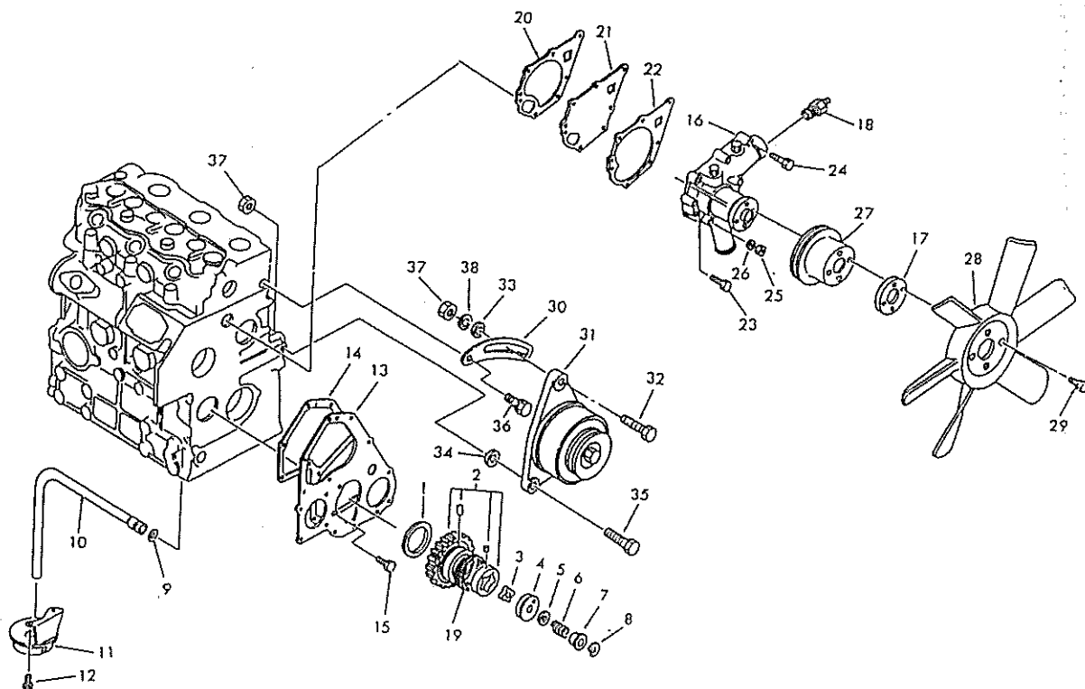
FIG.105 オイルポンプ, ウォーターポンプ OIL PUMP, WATER PUMP
