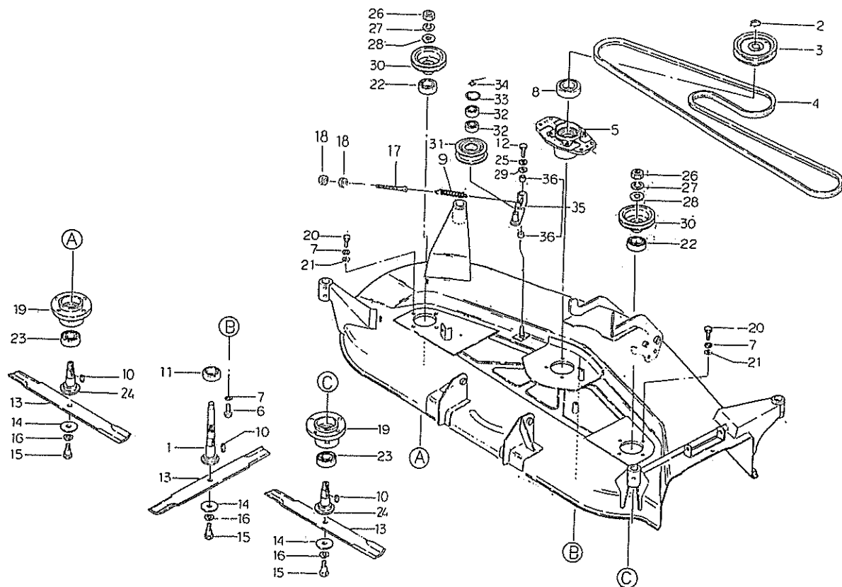
FIG.314 ブレード、プーリ BLADE, PULLEY : 60"
