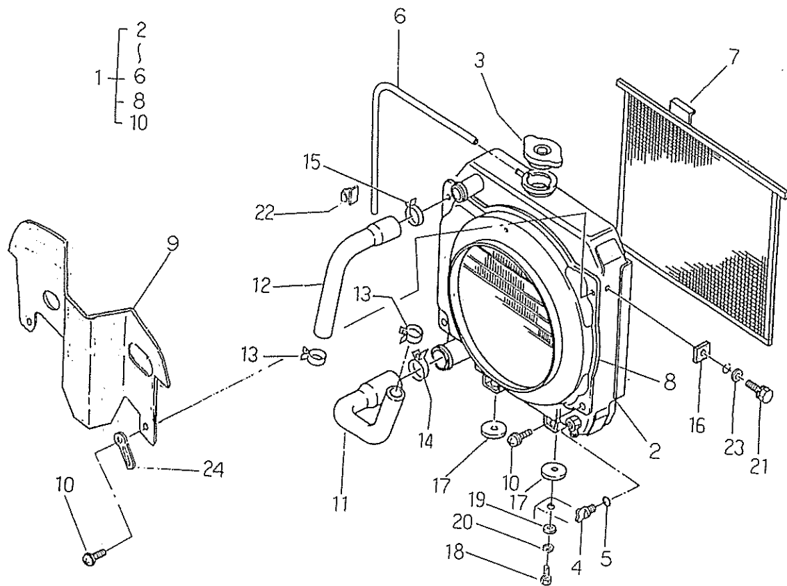
FIG.101 ラジエタ RADIATOR
