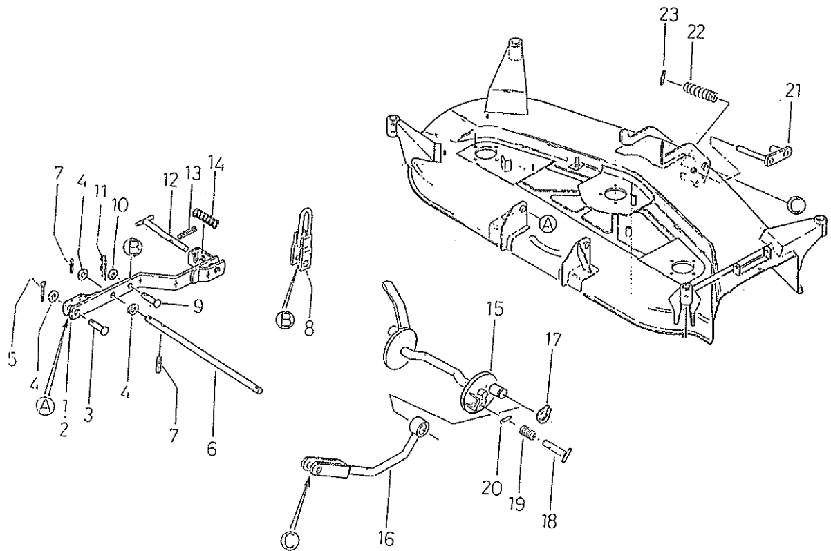
FIG.316 リンク LINK ; 60"
