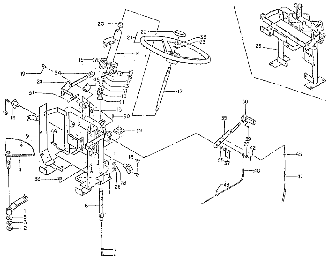
FIG.203 ステアリング STEERING ; MANUAL
