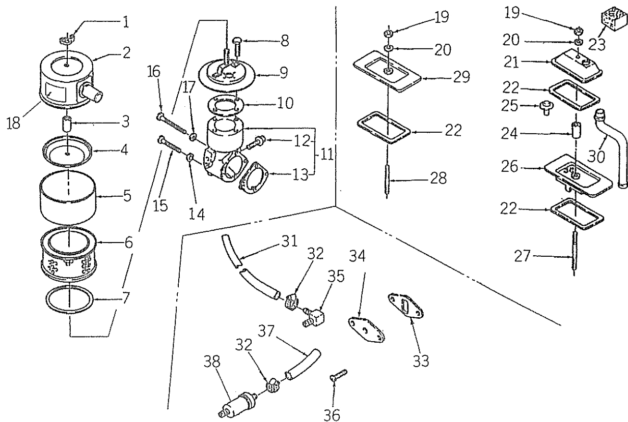
クリーナ、ブリーザ、フュエルフィルタ CLEANER, BREATHER, FUEL FILTER
