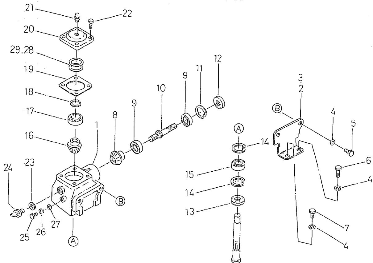
FIG.312 ギヤボックス GEAR BOX ; 60"
