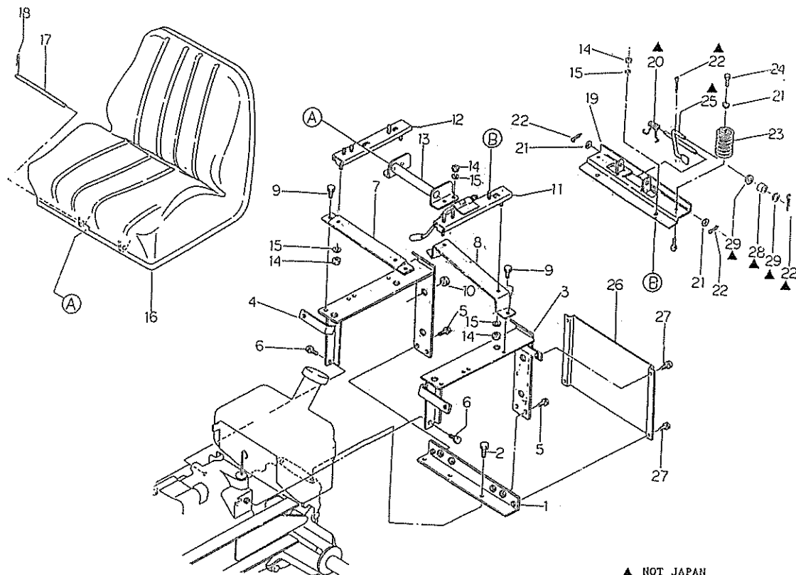
FIG.221 シート SEAT
