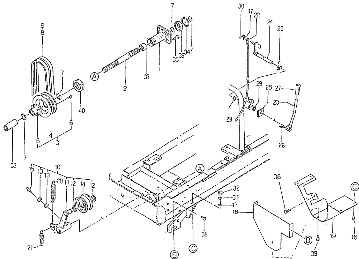
FIG.201 フロント P. T. O FRONT P. T. O
