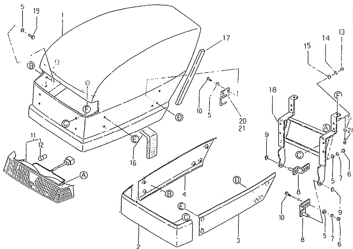
FIG.226 ボンネット BONNET
