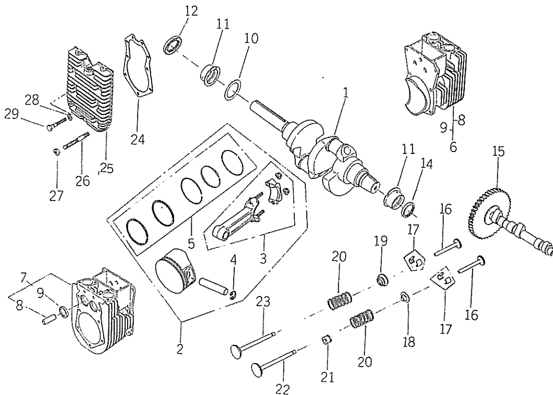
FIG.122 クランクシャフト, カムシャフト CRANKSHAFT, CAMSHAFT
