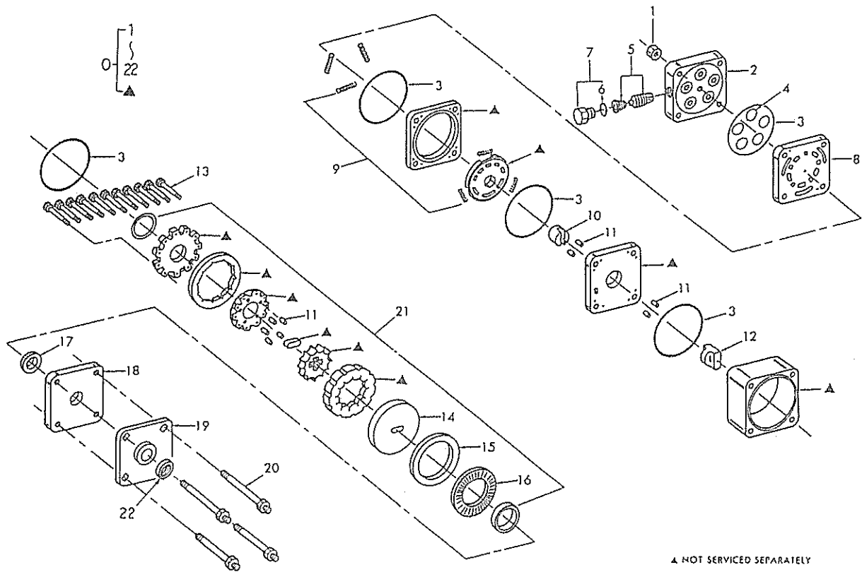
FIG.205 パワーステアリングパーツ POWER STEERING PARTS
