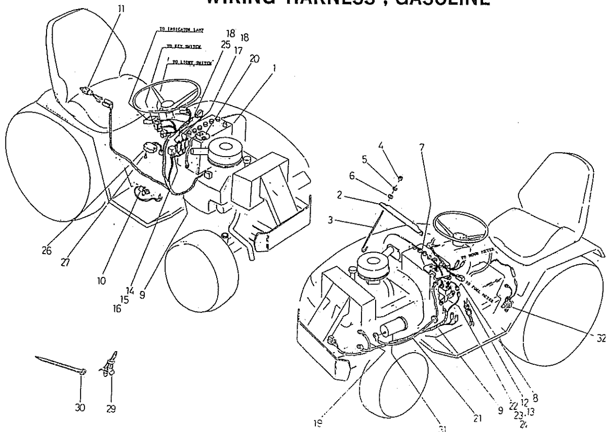
FIG.223 配線系統 WIRING HARNESS ; GASOLINE
