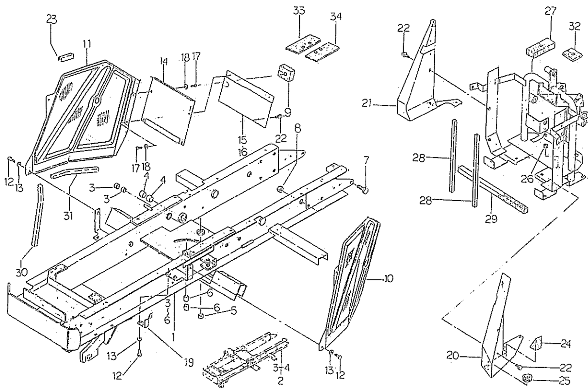
FIG.207 シャーシ, ダッシュボード CHASSIS, DASH BOARD ; DIESEL
