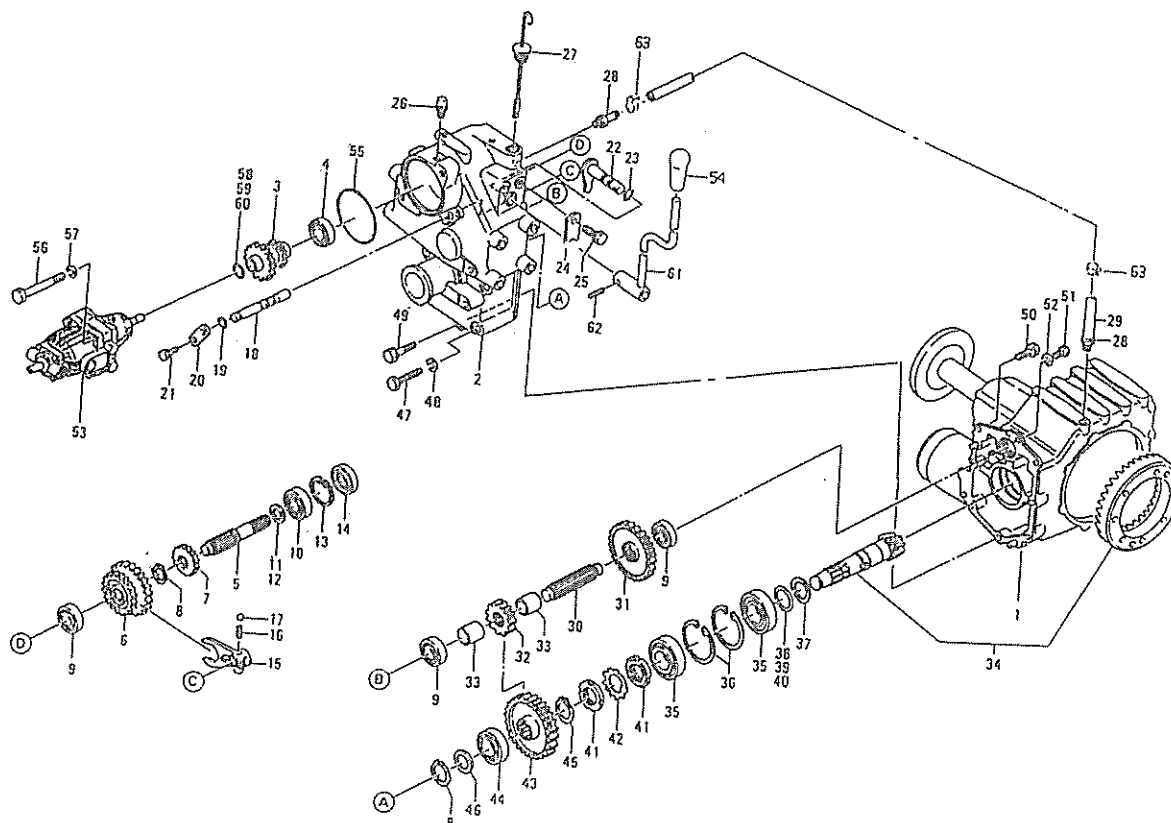
FIG.211 トランスミッション TRANSMISSION
