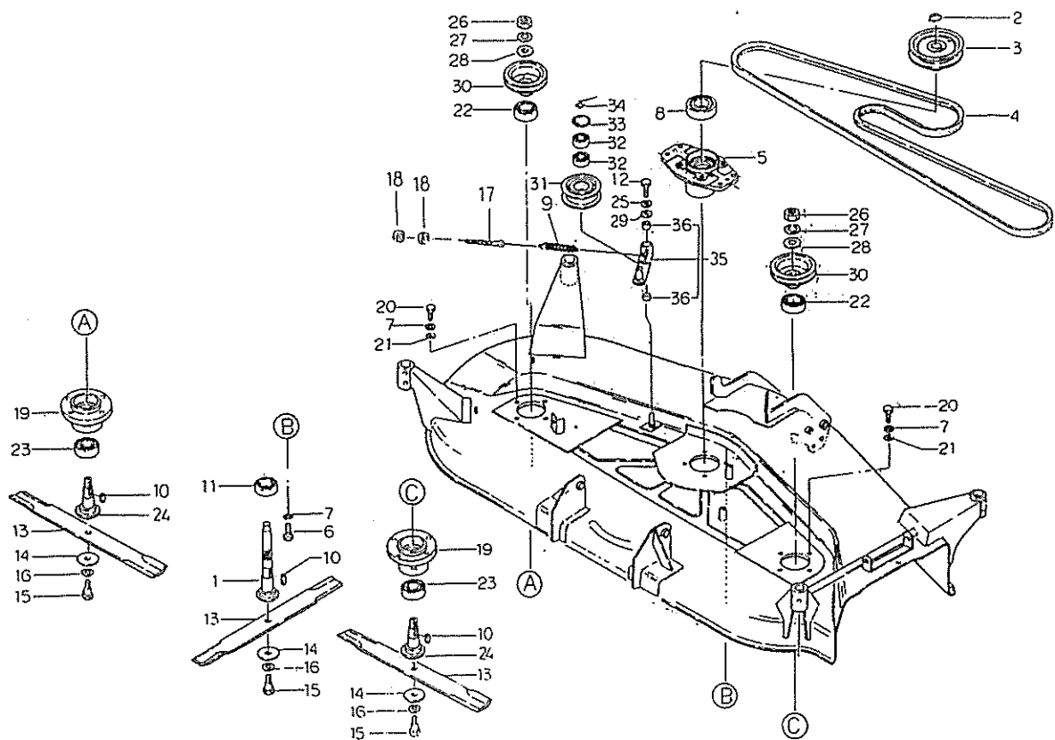
BLADE, PULLEY ; 60"
