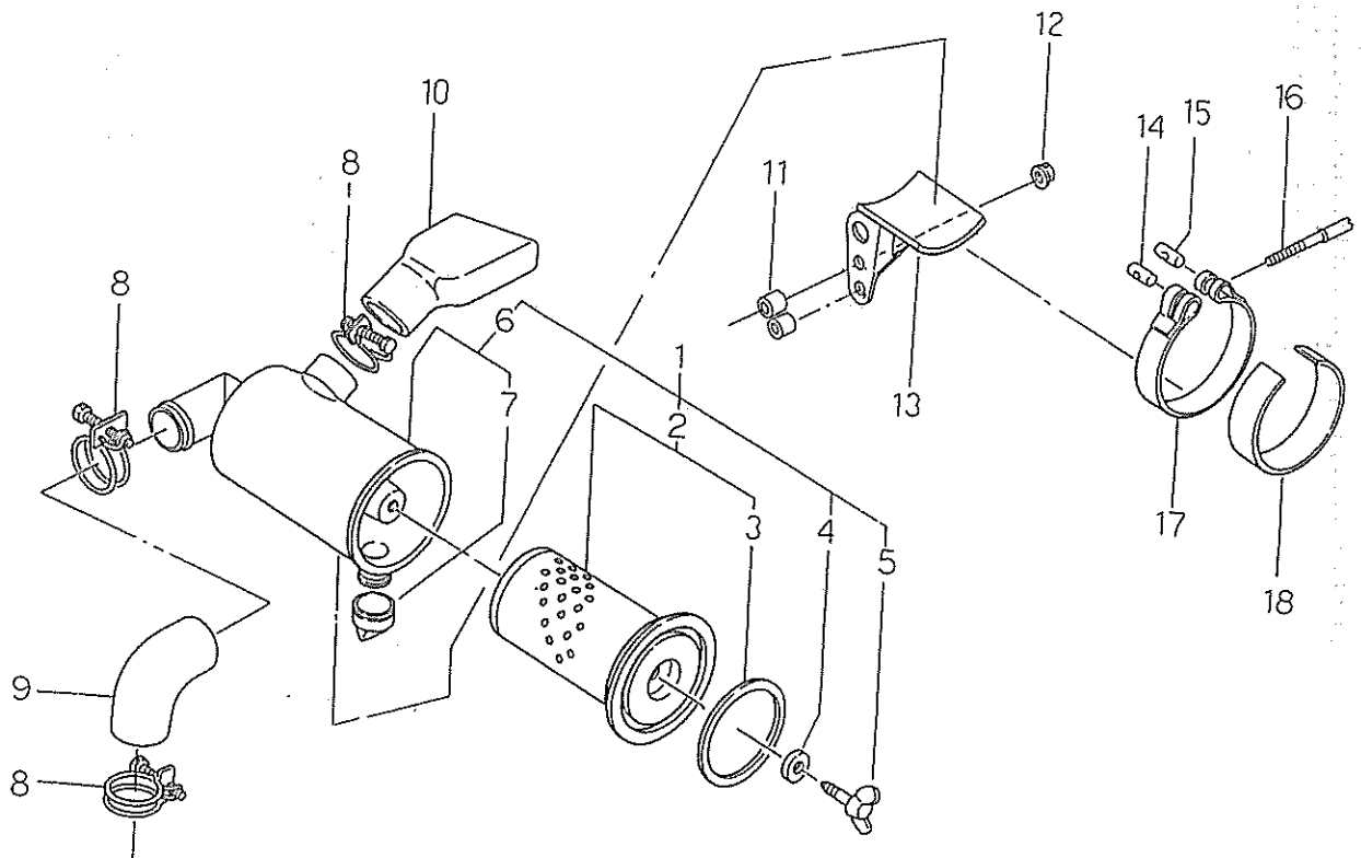
FIG.110 エヤクリーナ AIR CLEANER
