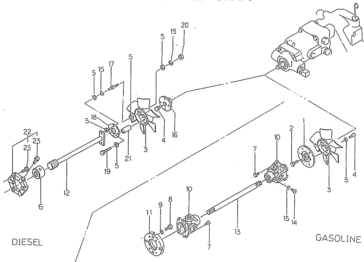
FIG.209 プロペラシャフト PROPELLER SHAFT
