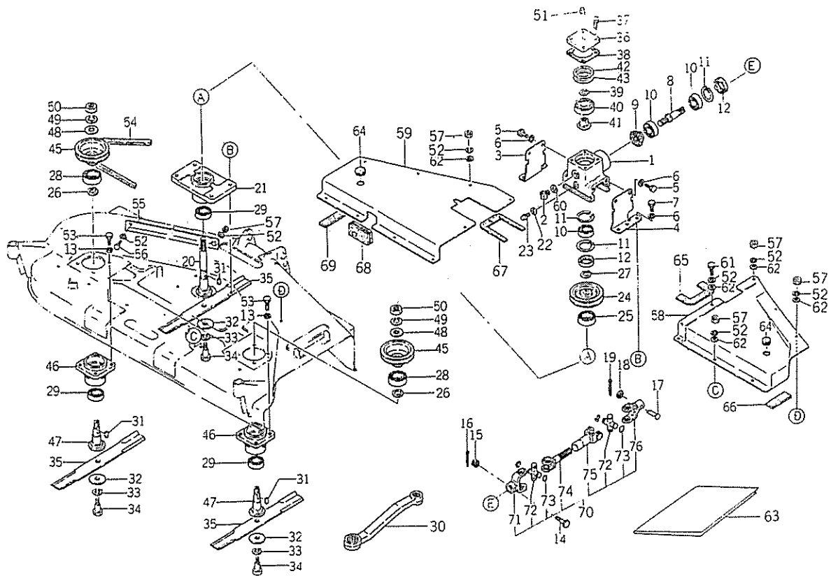
FIG.301 ギヤボックス, ブレード GEAR BOX, BLADE ; 44" & 48"
