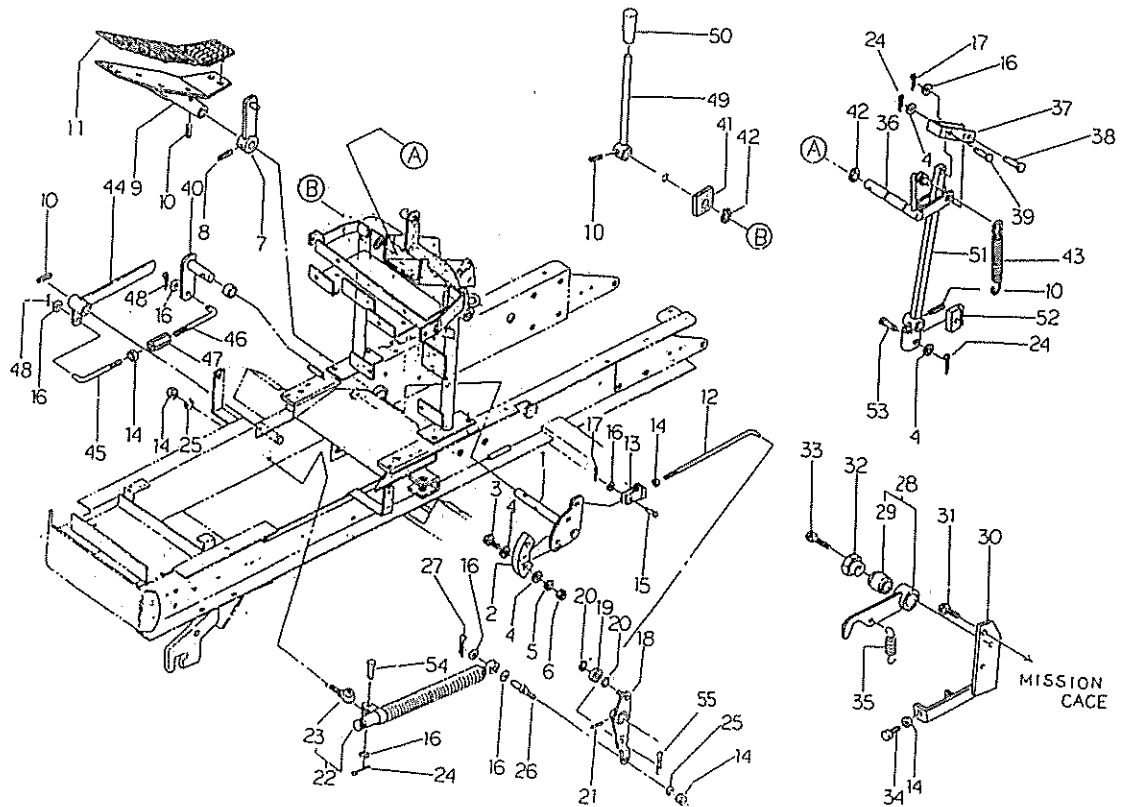
FIG.213 スピードコントロール SPEED CONTROL
