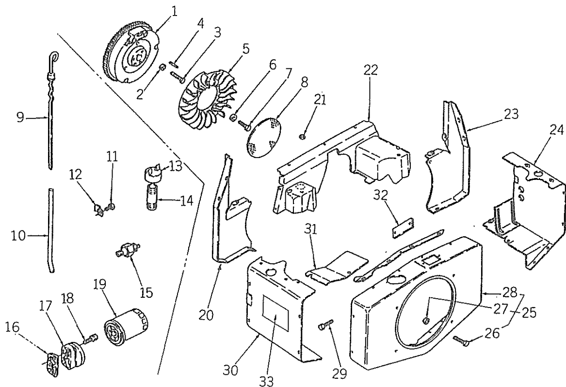
FIG.124 フライホイール, オイルフィルタ, クーリングカバー FLY WHEEL, OIL FILTER, COOLING COVER
