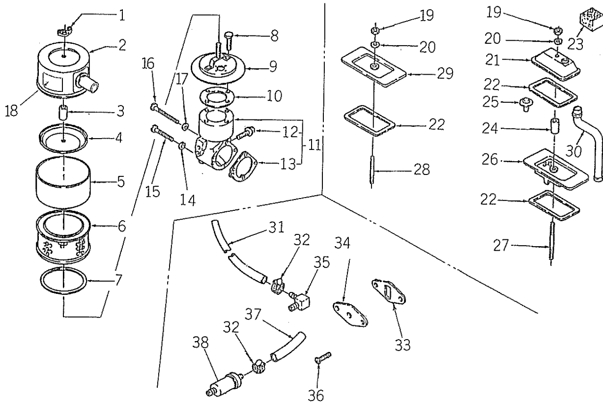
FIG.125 クリーナ、ブリーザ、フュエルフィルタ CLEANER, BREATHER, FUEL FILTER
