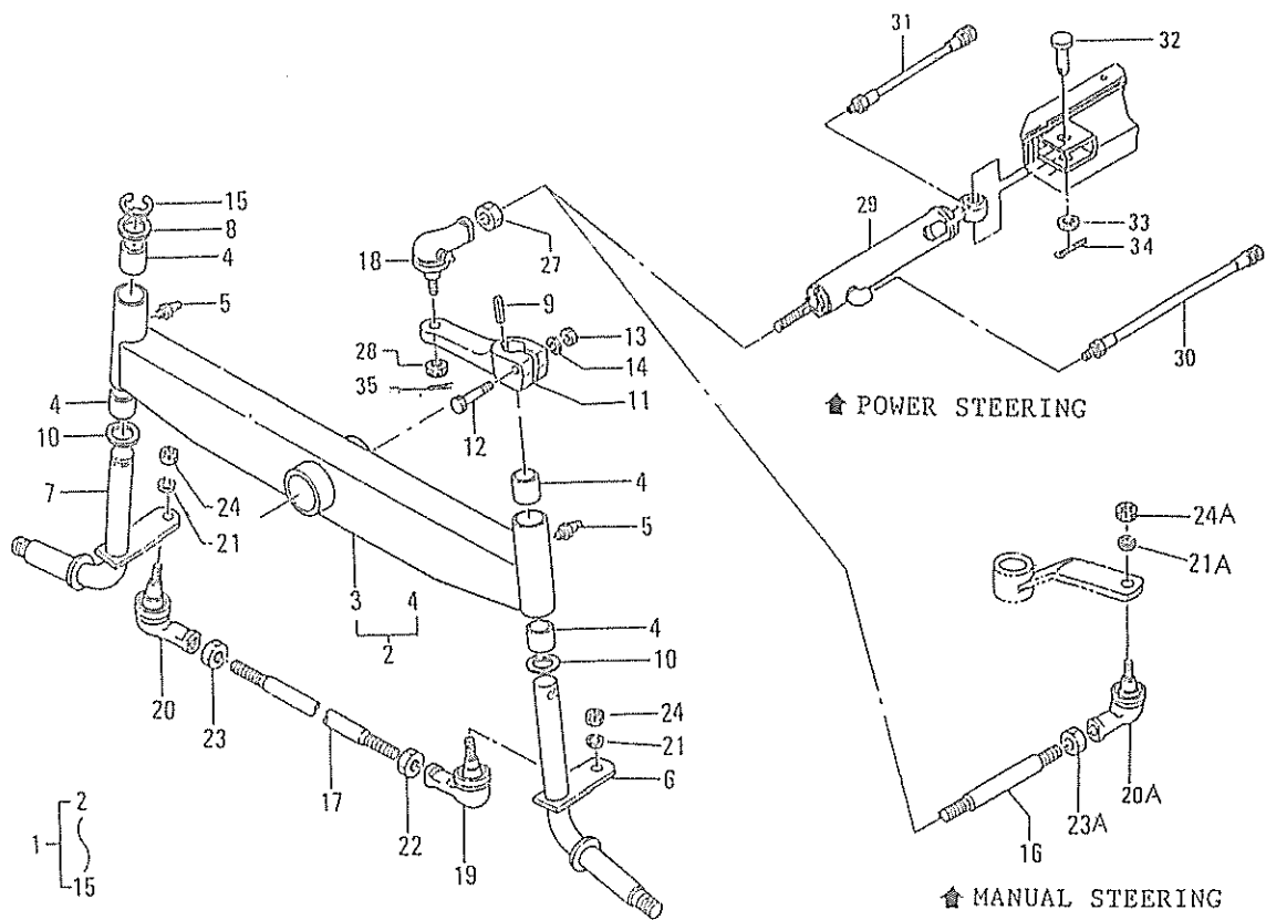
フロントアクスル FRONT AXLE
