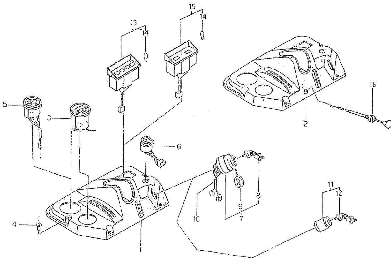
インスツルメントパネル INSTRUMENT PANEL
