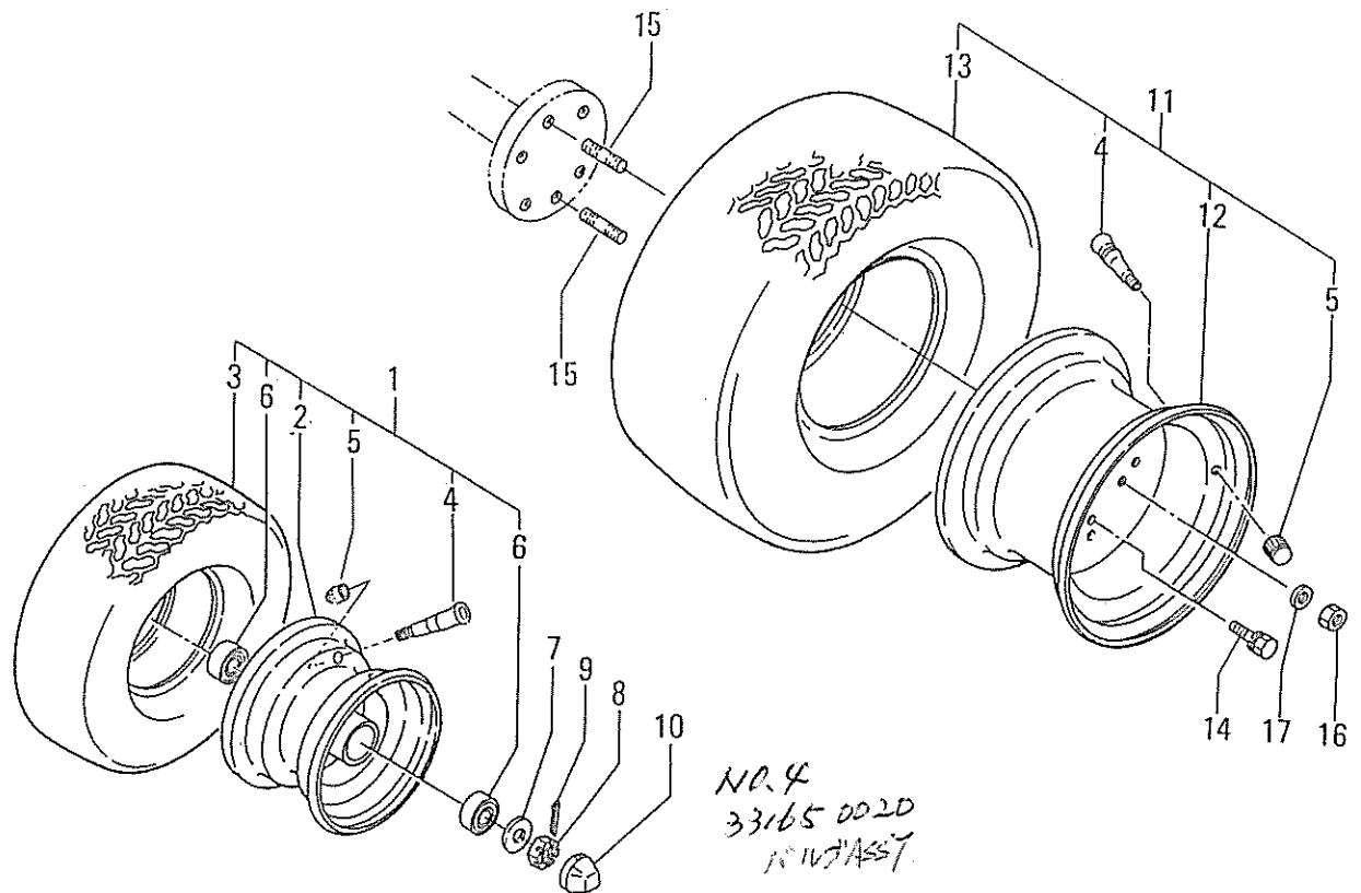
FIG.225 フロントホイール, リヤホイール FRONT WHEELS, REAR WHEELS
