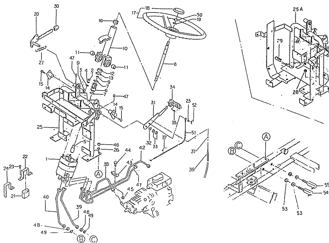
FIG.204 ステアリング STEERING ; POWER
