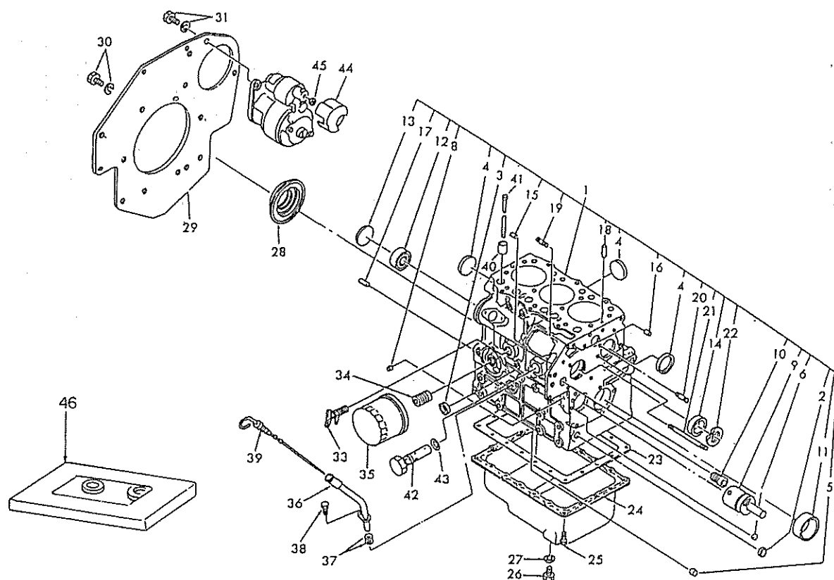
FIG.102 シリンダブロック CYLINDER BLOCK
