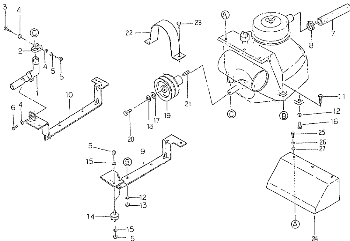
FIG.128 エンジンマウント ENGINE MOUNT ; GASOLINE
