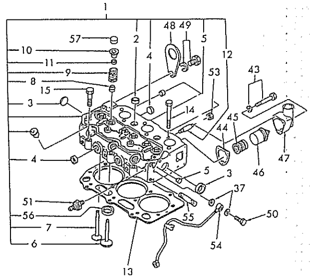
FIG.103 シリンダヘッド CYLINDER HEAD
