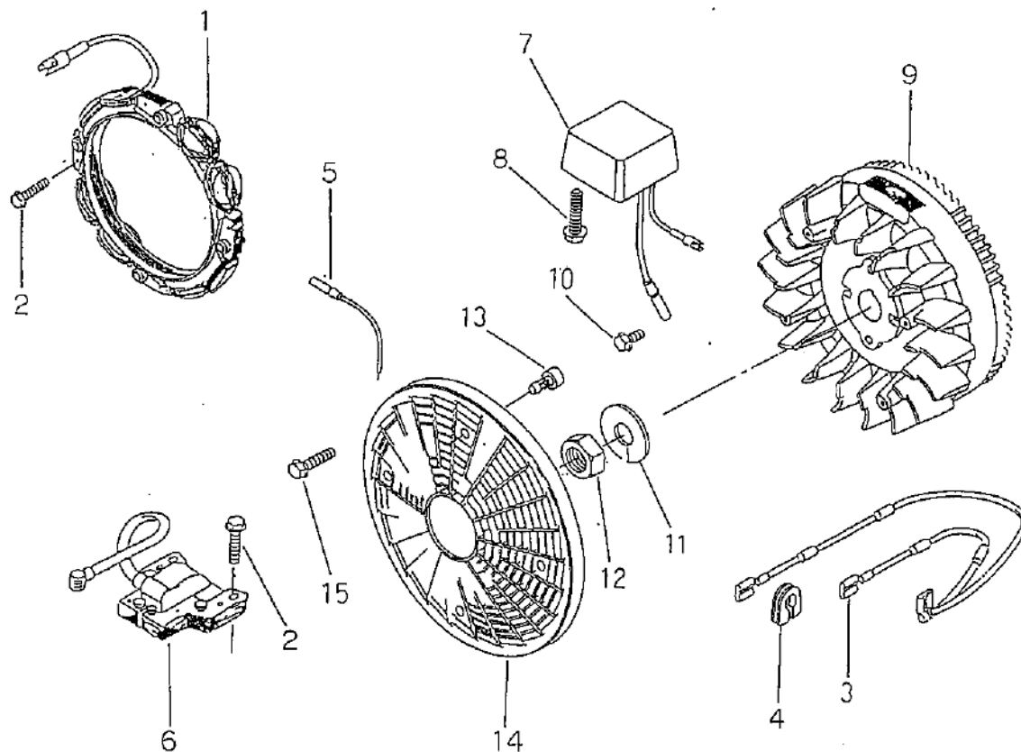
フライホイール, マグネット FLY WHEEL, MAGNET
