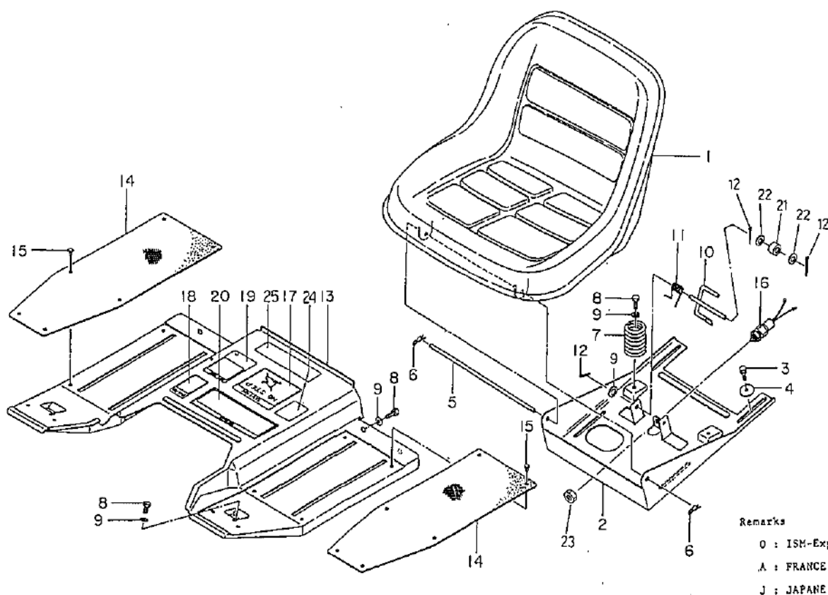
FIG.213 シート, ステップ SEAT, STEPS
