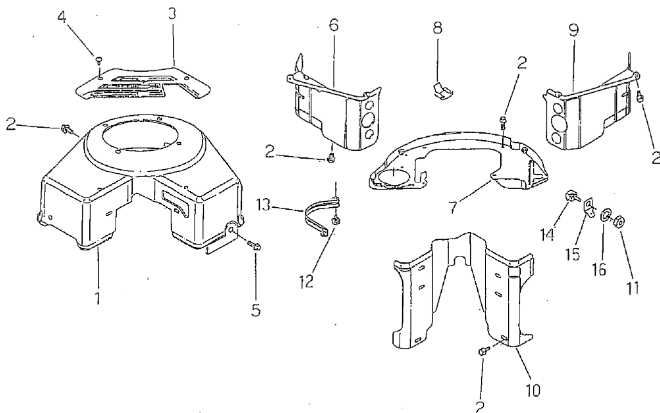
クーリングカバー, マフラー COOLING COVER, MUFFLER
