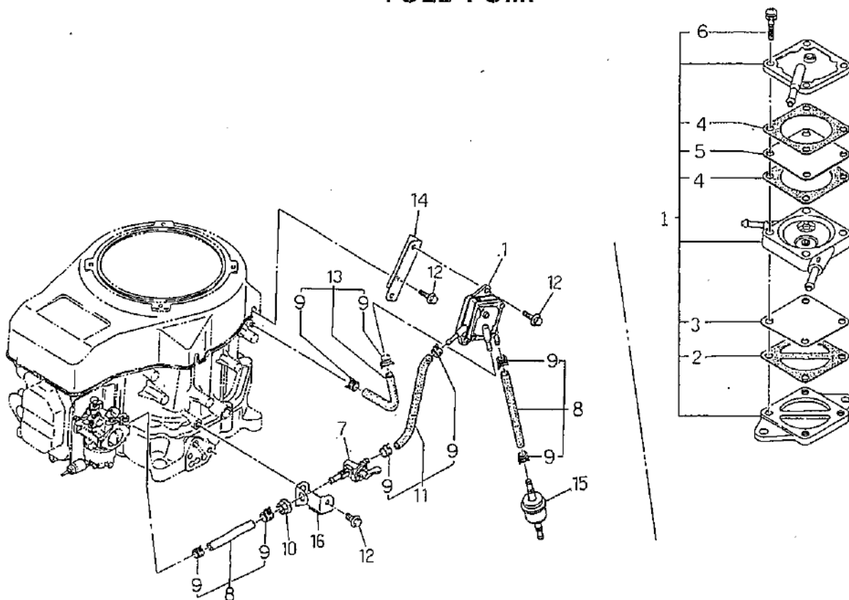
FIG.106 フューエルポンプ FUEL PUMP
