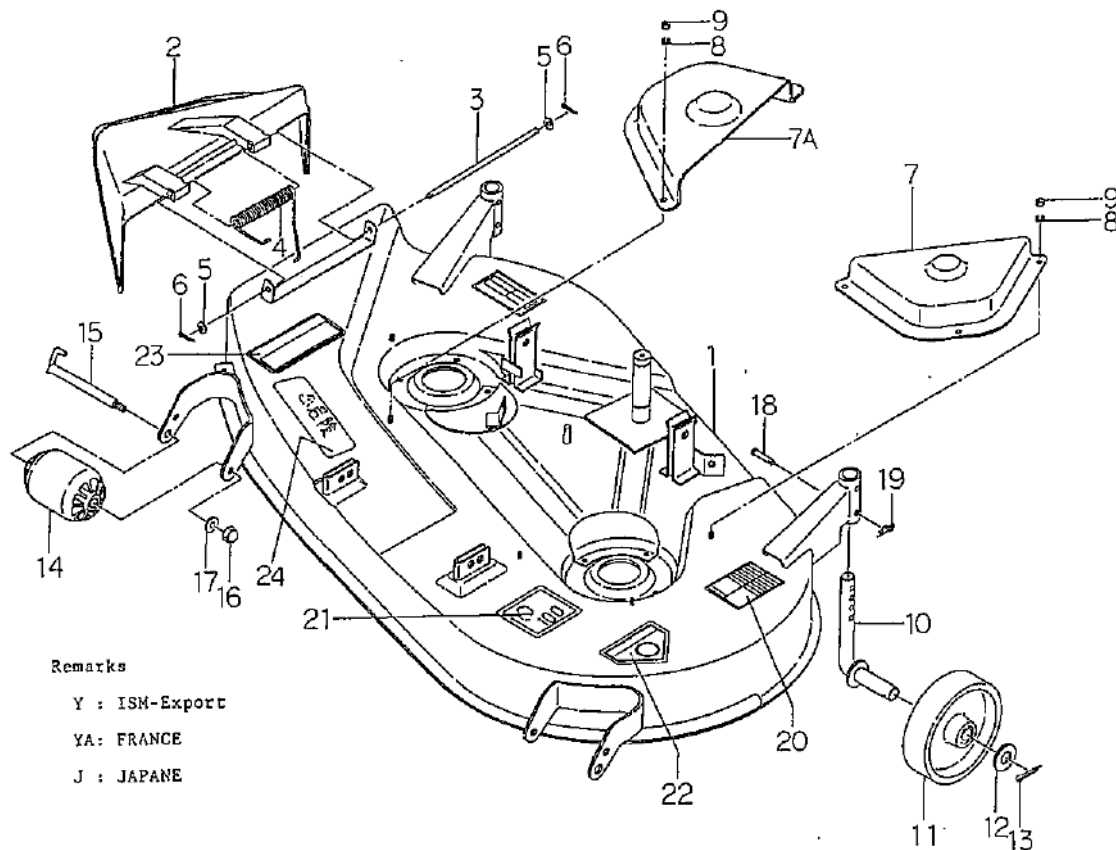
FIG.301 デッキ, カバー MOWER DECK, COVER ; MM 40
