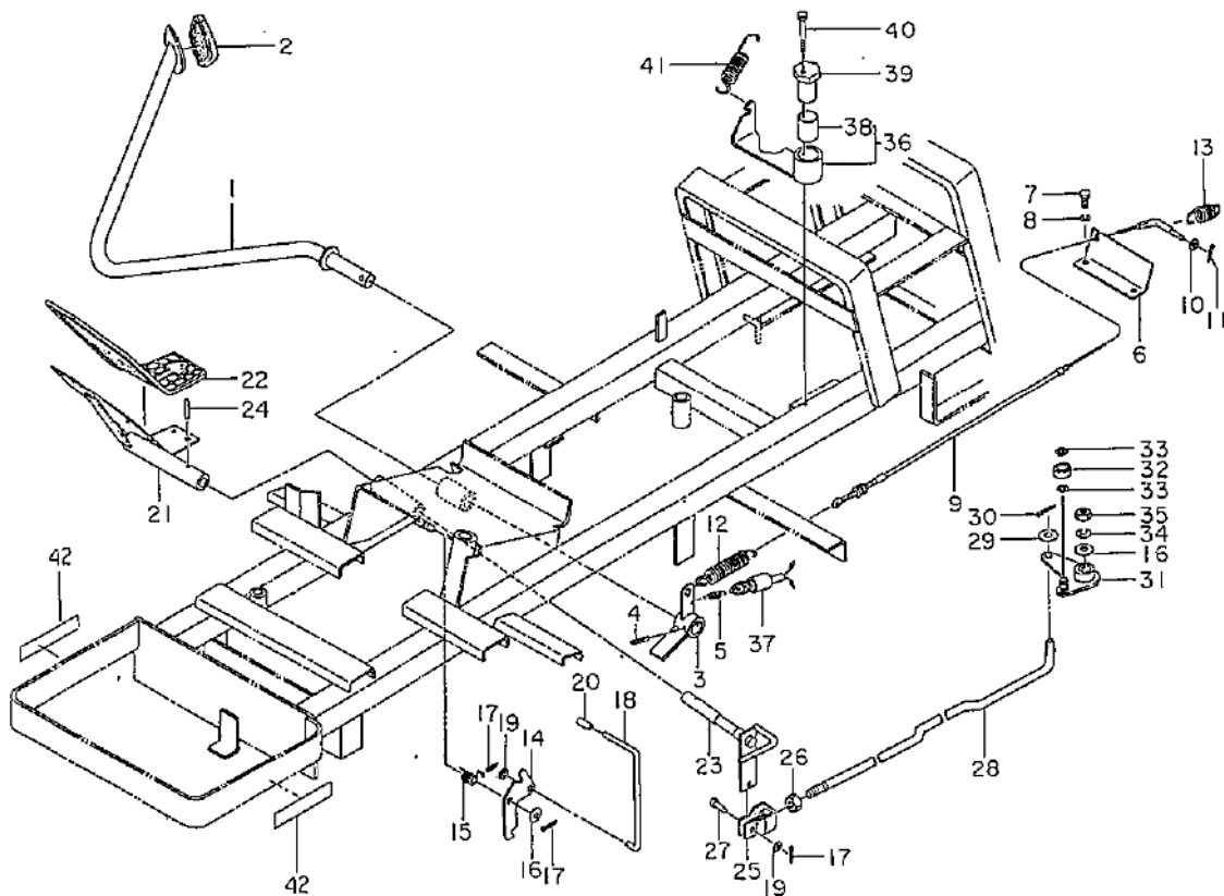
ブレーキ, ペダル BRAKE, PEDALS
