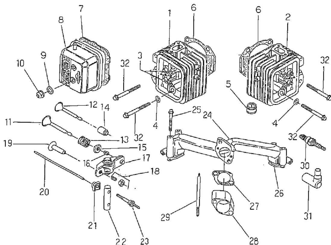
FIG.113 シリンダヘッド CYLINDER HEAD
