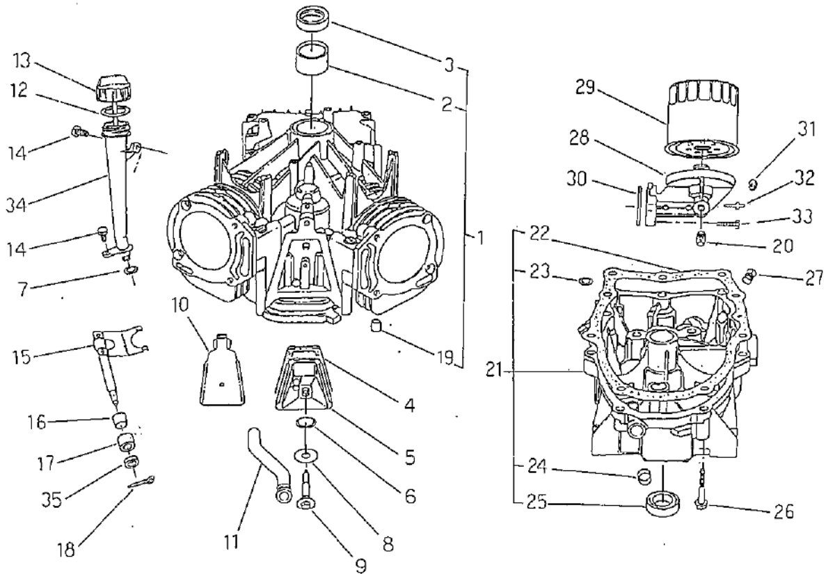
FIG.111 シリンダブロック CYLINDER BLOCK
