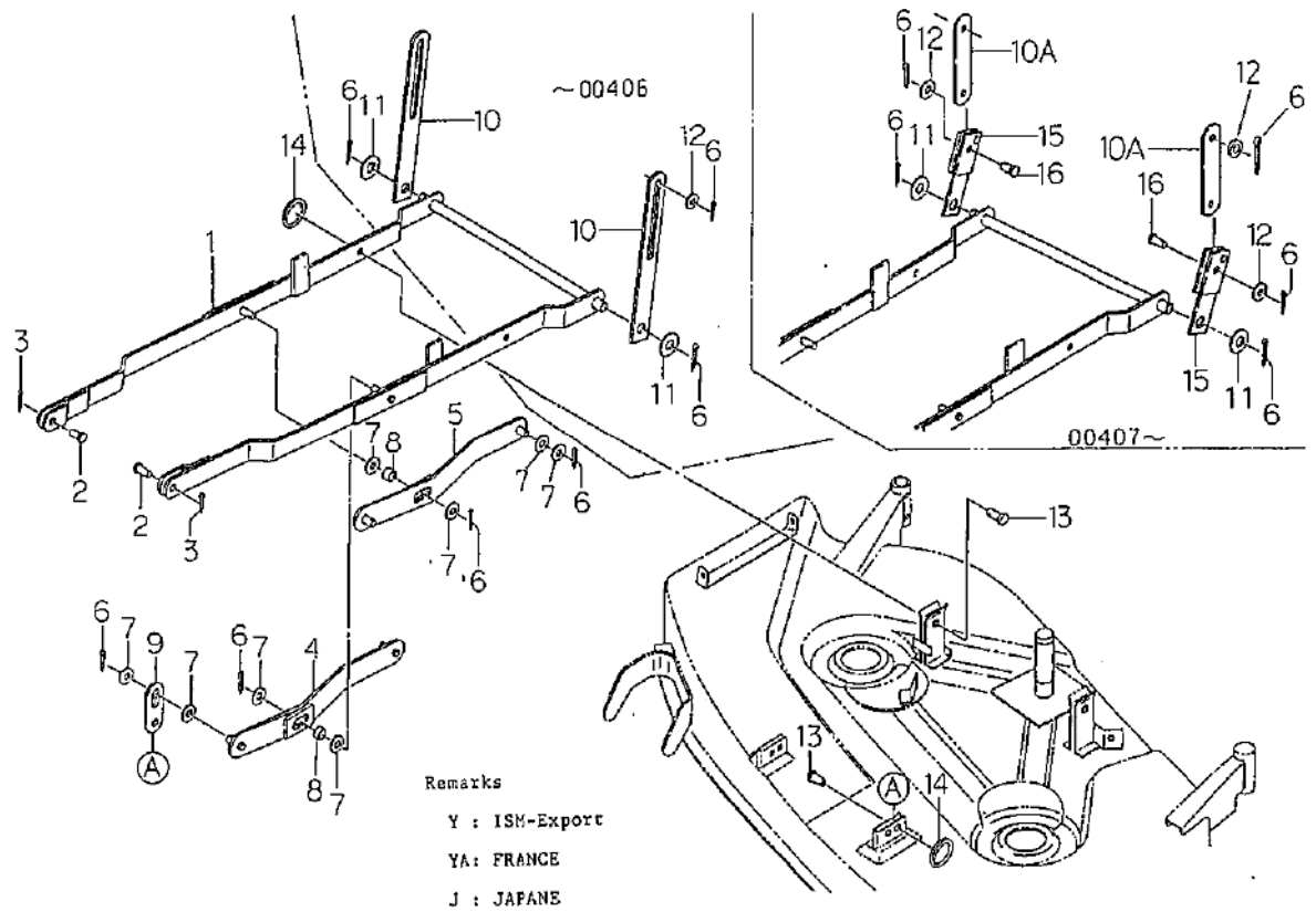
FIG.303 リンク LINK ; MM 40
