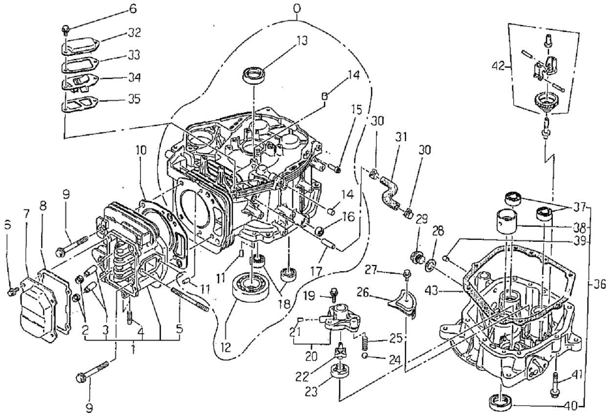
クランクケース CRANK CASE
