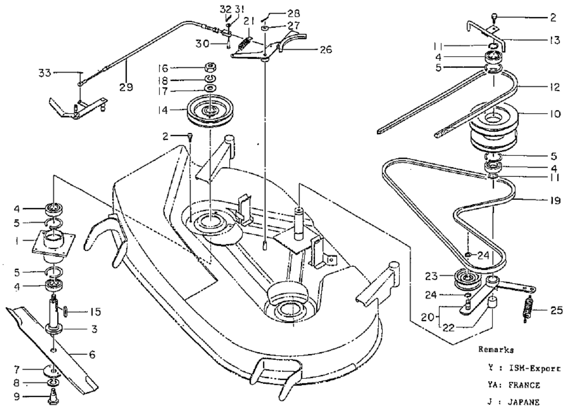
FIG.302 プーリ, テンション PULLEY, TENSION ; MM 40
