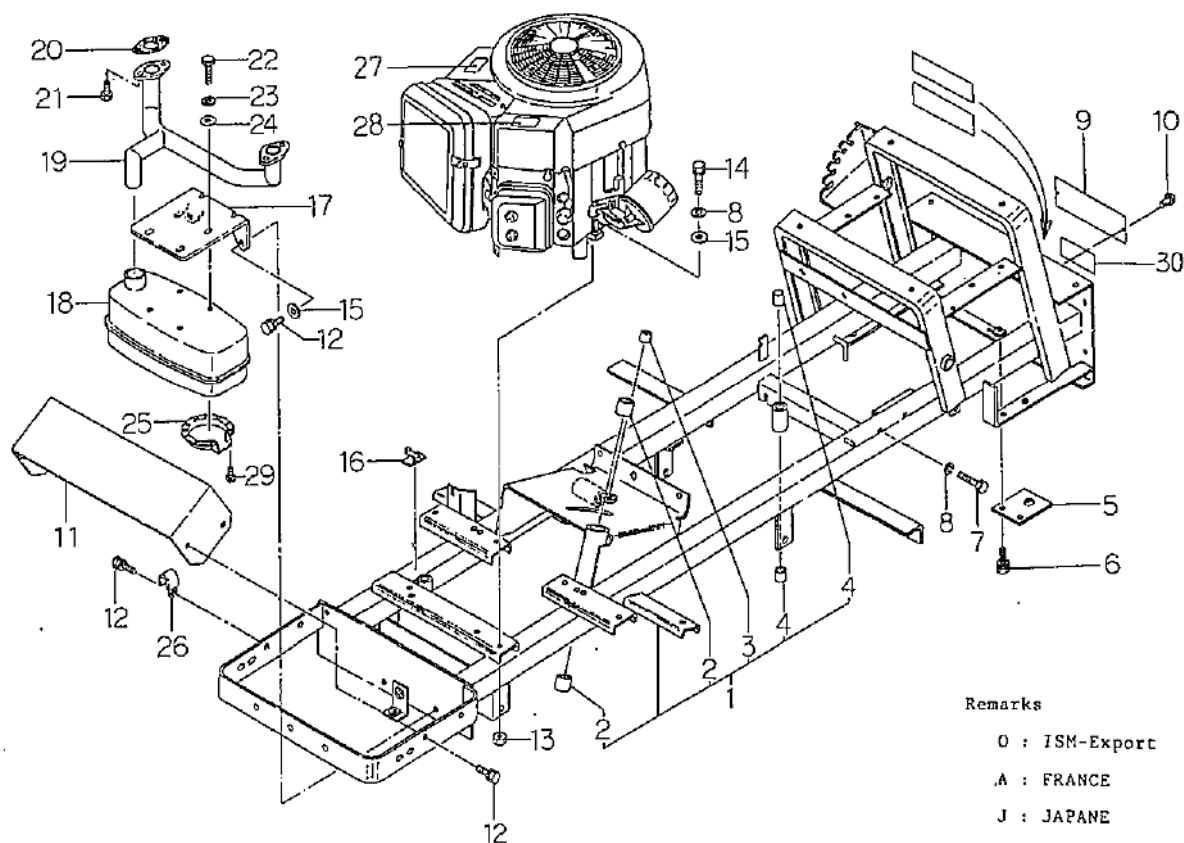
FIG.202 シャーシ, マフラ CHASSIS MUFFLER ; LT 16
