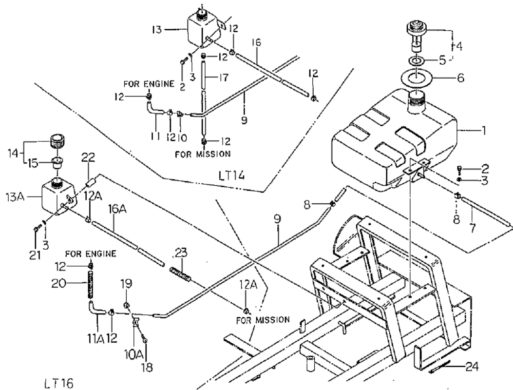
FIG.206 フューエルタンク, オイルタンク FUEL TANK, OIL TANK
