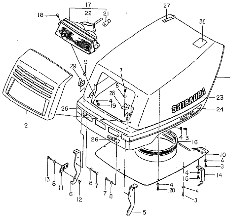
ボンネット BONNET
