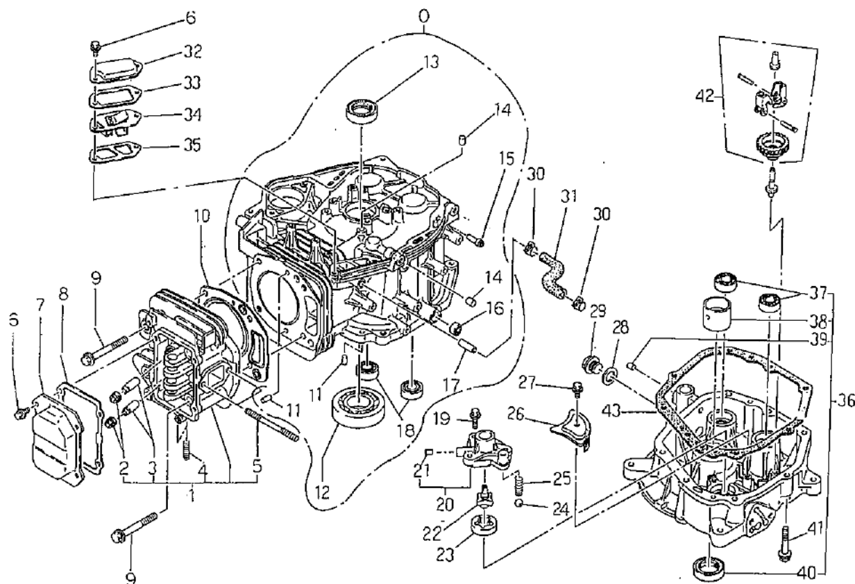
FIG.101 クランクケース CRANK CASE
