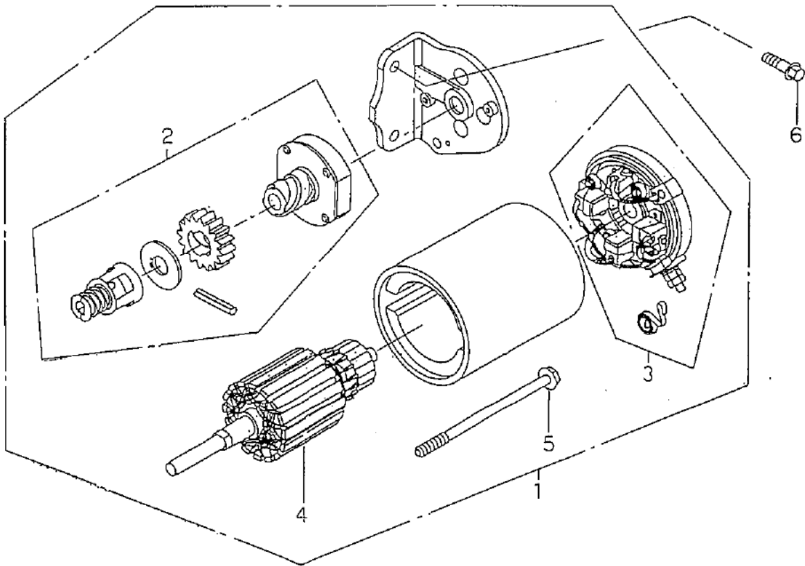
スターティングモータ STARTING MOTOR
