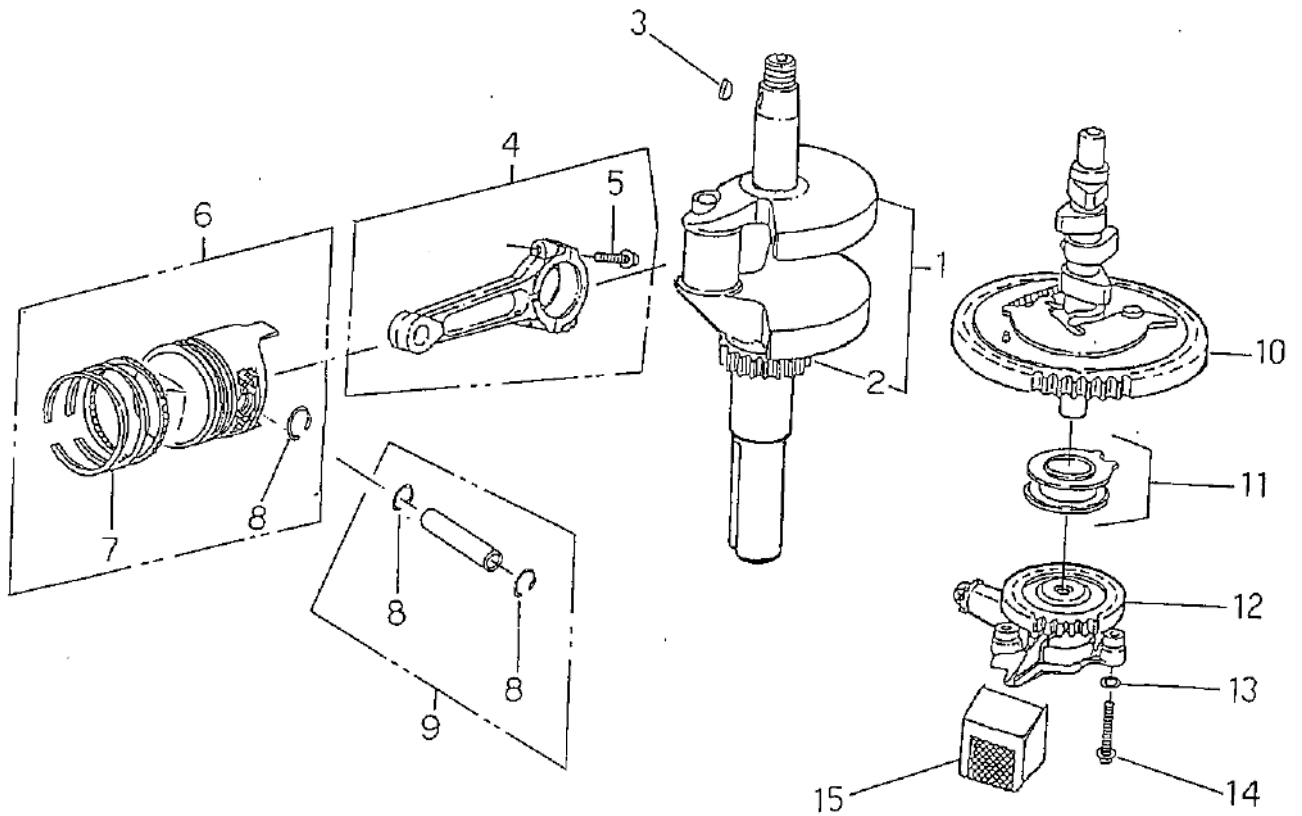
クランクシャフト, ピストン CRANKSHAFT, PISTON
