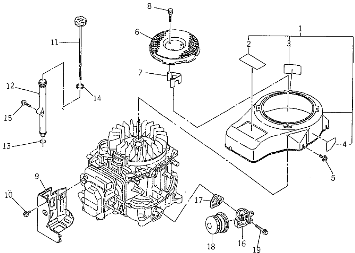
クーリングカバー, オイルフィルタ COOLING COVER, OIL FILTER
