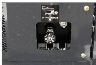
コンベアベルトのスピードはダイヤルを回すだけで簡単に調整できます。
