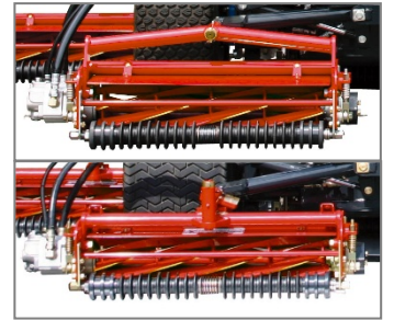
モアは、横軸タイプ（写真上5枚刃・7枚刃）と縦軸タイプ（写真下9枚刃）があります。使うシーンによって選択できます。
