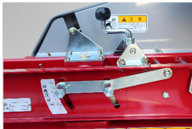
刈高の調整は、ロータリーデッキ上部にあるハンドルを回し、目盛りに合わせることで調整できます。
