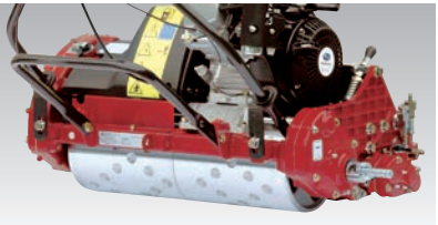
D (ディンプル)ドラム
