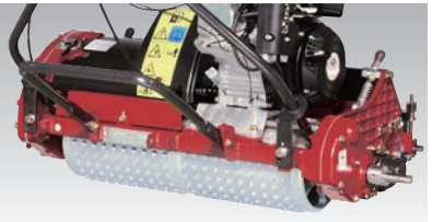
ラグドラム (LM66TB)
