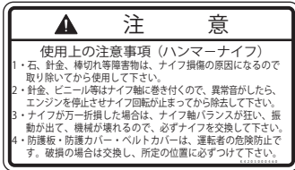
K4205000460 ハンマーナイフ点検事項
